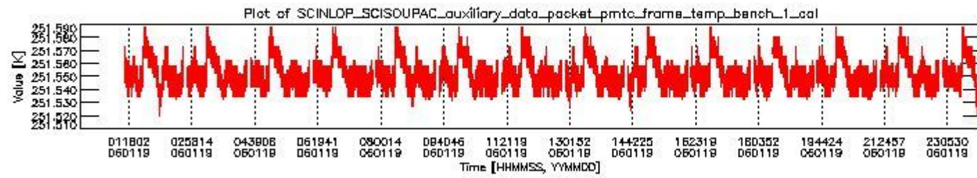
sciamachy_daily_report_level0_PFHS_5_35_N_20060119_0.PNG
