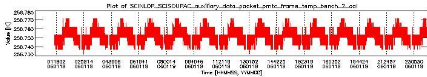
sciamachy_daily_report_level0_PFHS_5_35_N_20060119_1.PNG
