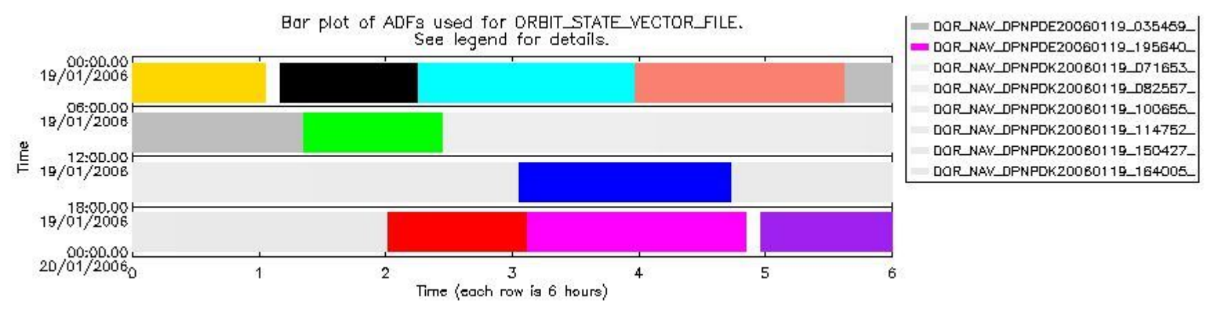
sciamachy_daily_report_level0_PFHS_5_35_N_20060119_6.PNG
