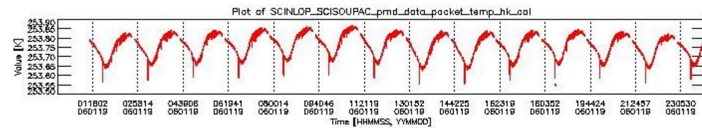
sciamachy_daily_report_level0_PFHS_5_35_N_20060119_3.PNG
