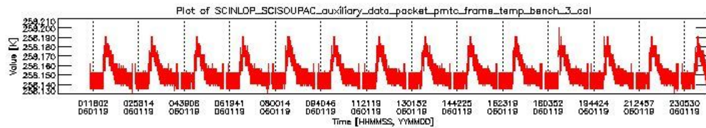
sciamachy_daily_report_level0_PFHS_5_35_N_20060119_2.PNG
