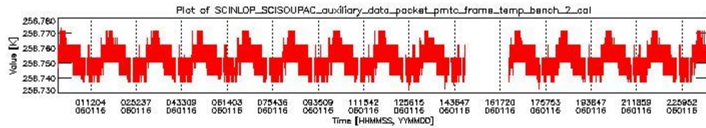
sciamachy_daily_report_level0_PFHS_5_35_N_20060116_1.PNG
