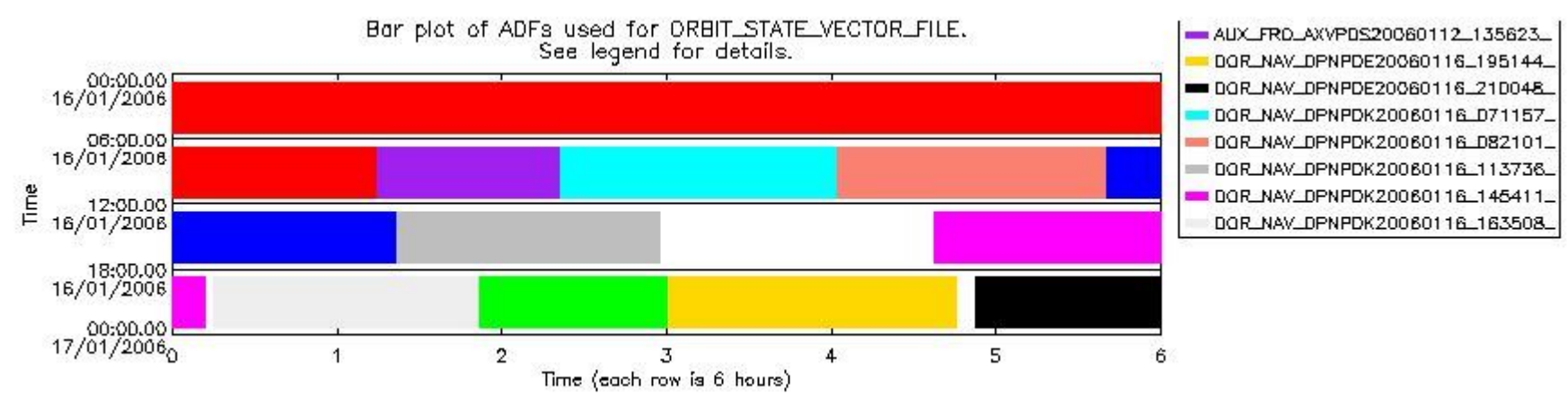
sciamachy_daily_report_level0_PFHS_5_35_N_20060116_6.PNG
