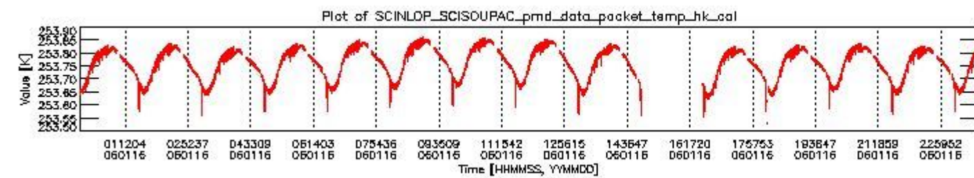
sciamachy_daily_report_level0_PFHS_5_35_N_20060116_3.PNG
