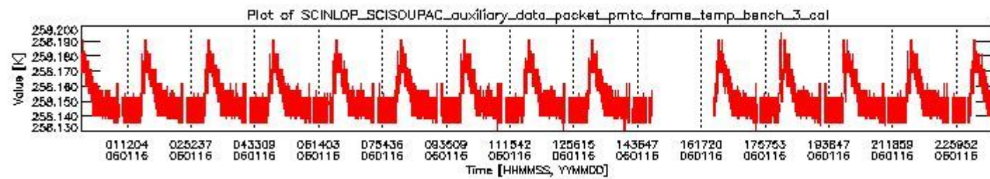
sciamachy_daily_report_level0_PFHS_5_35_N_20060116_2.PNG
