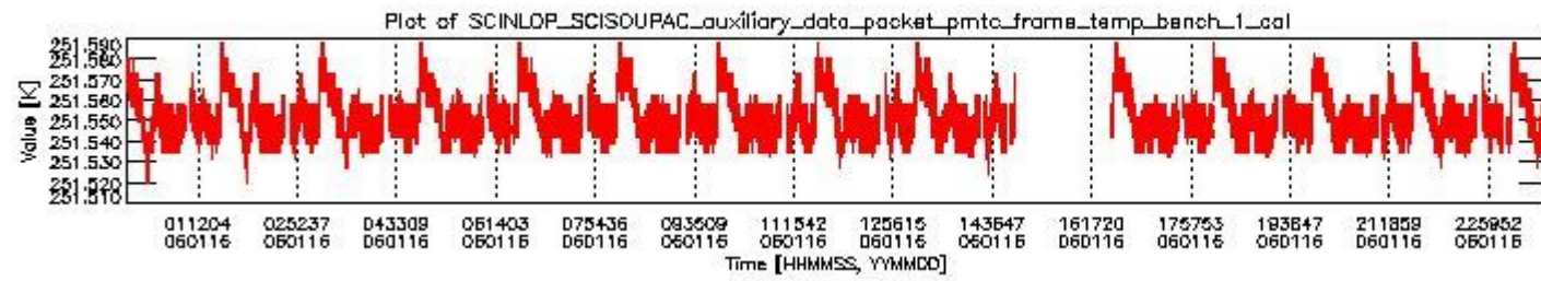
sciamachy_daily_report_level0_PFHS_5_35_N_20060116_0.PNG
