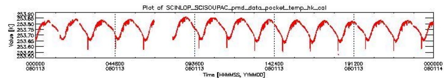
sciamachy_daily_report_level0_PFHS_5_35_N_20060113_3.PNG
