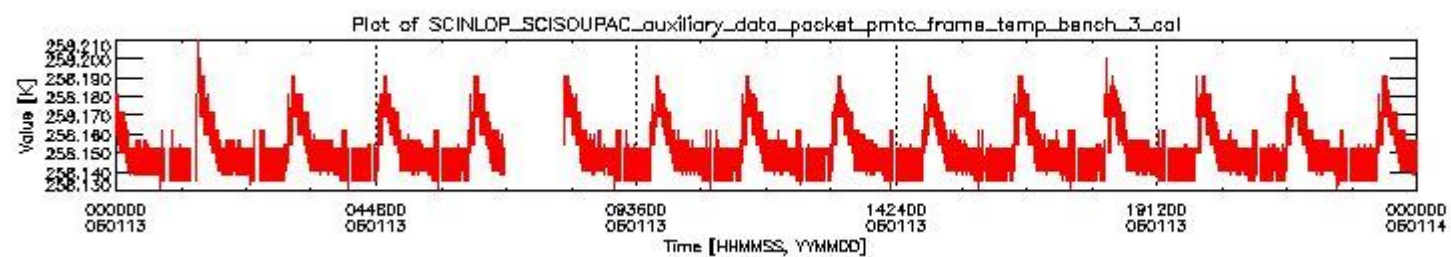
sciamachy_daily_report_level0_PFHS_5_35_N_20060113_2.PNG
