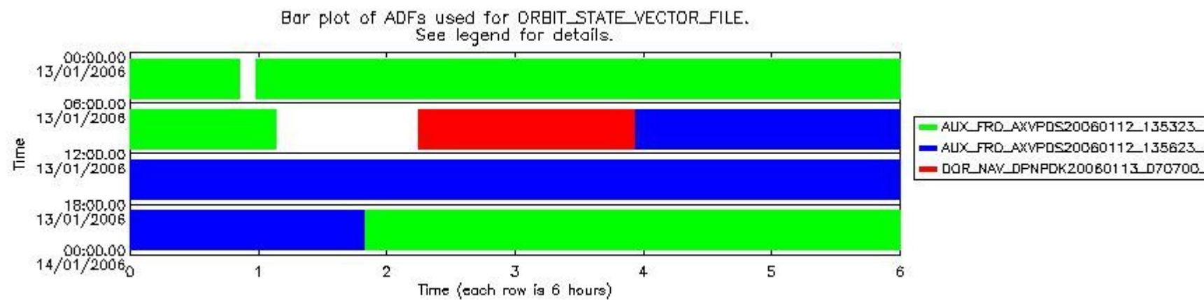
sciamachy_daily_report_level0_PFHS_5_35_N_20060113_6.PNG
