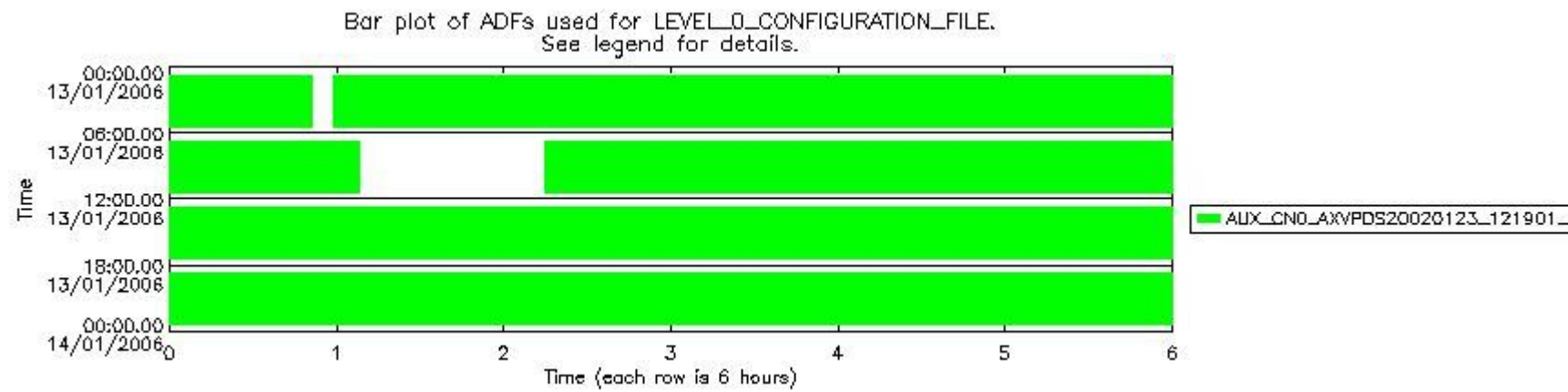
sciamachy_daily_report_level0_PFHS_5_35_N_20060113_5.PNG
