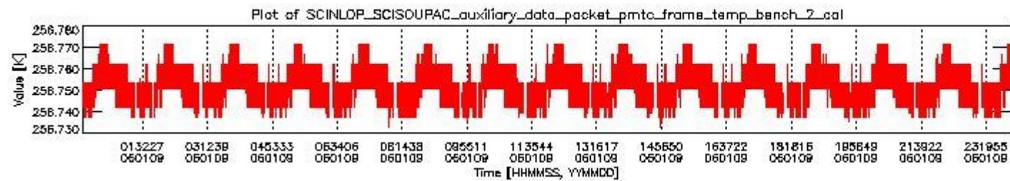
sciamachy_daily_report_level0_PFHS_5_34_N_20060109_1.PNG
