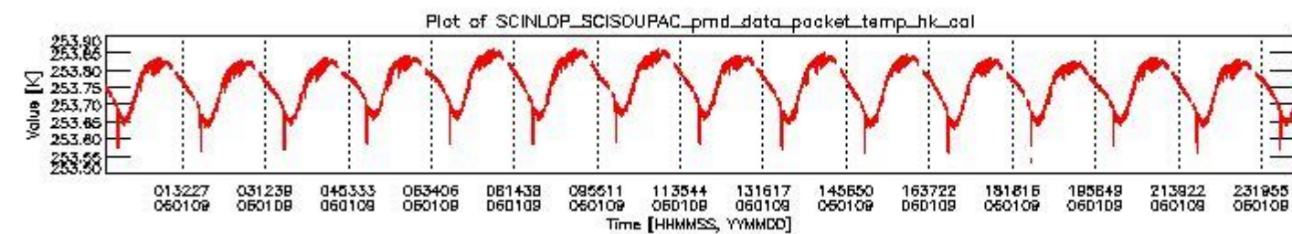
sciamachy_daily_report_level0_PFHS_5_34_N_20060109_3.PNG
