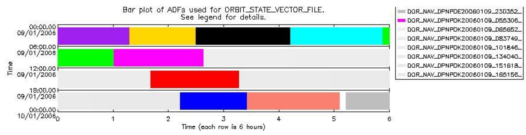
sciamachy_daily_report_level0_PFHS_5_34_N_20060109_6.PNG
