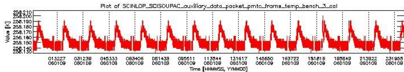
sciamachy_daily_report_level0_PFHS_5_34_N_20060109_2.PNG
