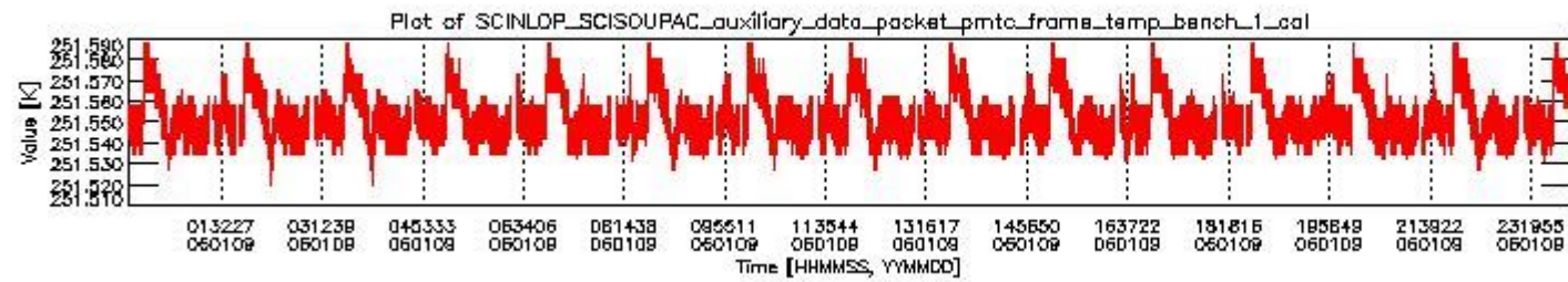
sciamachy_daily_report_level0_PFHS_5_34_N_20060109_0.PNG
