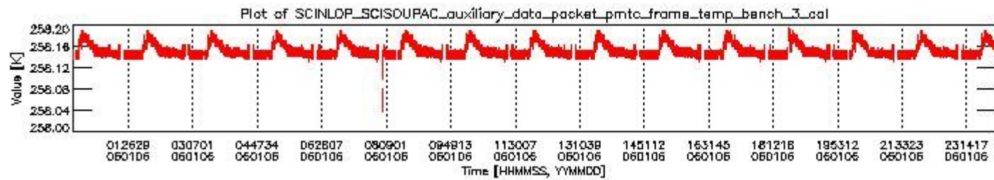
sciamachy_daily_report_level0_PFHS_5_34_N_20060106_2.PNG
