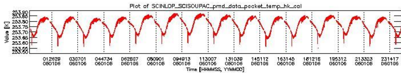
sciamachy_daily_report_level0_PFHS_5_34_N_20060106_3.PNG
