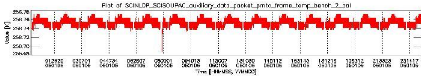
sciamachy_daily_report_level0_PFHS_5_34_N_20060106_1.PNG
