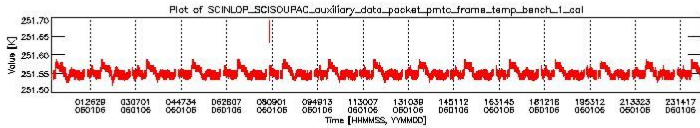
sciamachy_daily_report_level0_PFHS_5_34_N_20060106_0.PNG
