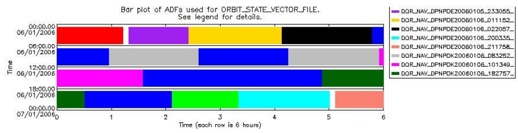
sciamachy_daily_report_level0_PFHS_5_34_N_20060106_6.PNG
