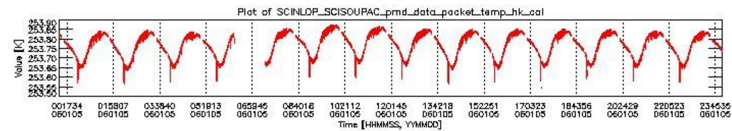
sciamachy_daily_report_level0_PFHS_5_34_N_20060105_3.PNG
