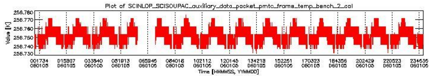
sciamachy_daily_report_level0_PFHS_5_34_N_20060105_1.PNG
