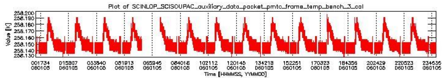
sciamachy_daily_report_level0_PFHS_5_34_N_20060105_2.PNG
