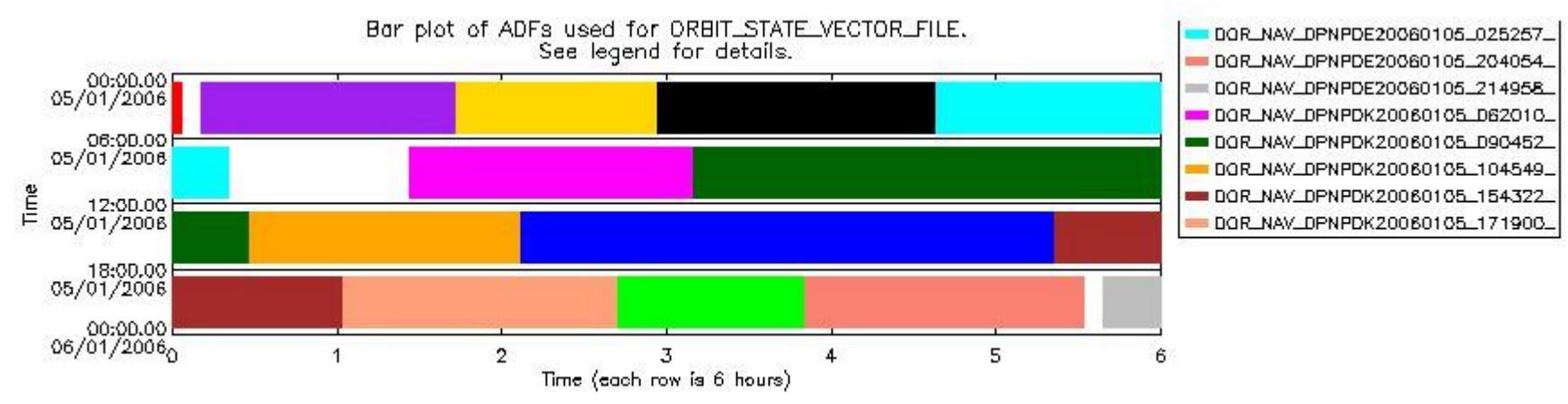
sciamachy_daily_report_level0_PFHS_5_34_N_20060105_6.PNG
