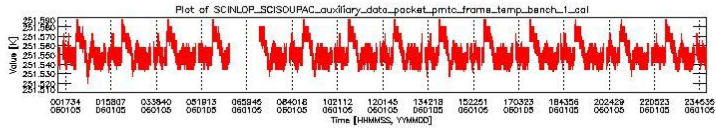
sciamachy_daily_report_level0_PFHS_5_34_N_20060105_0.PNG
