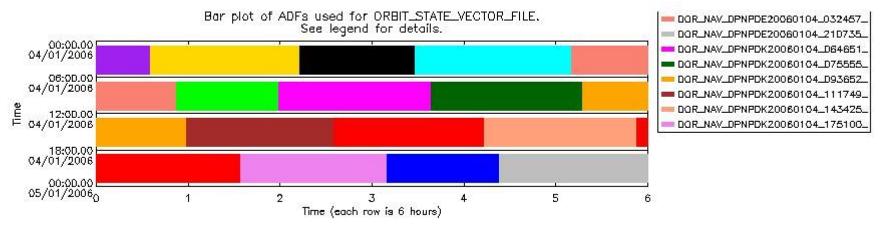
sciamachy_daily_report_level0_PFHS_5_34_N_20060104_6.PNG
