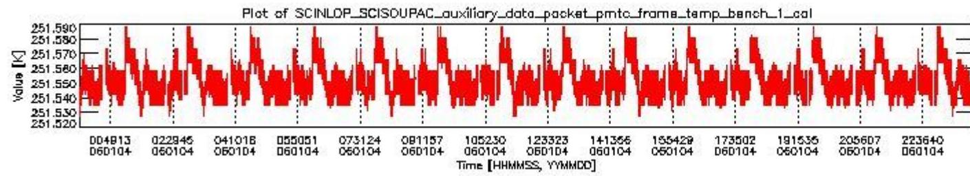
sciamachy_daily_report_level0_PFHS_5_34_N_20060104_0.PNG
