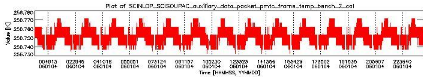
sciamachy_daily_report_level0_PFHS_5_34_N_20060104_1.PNG
