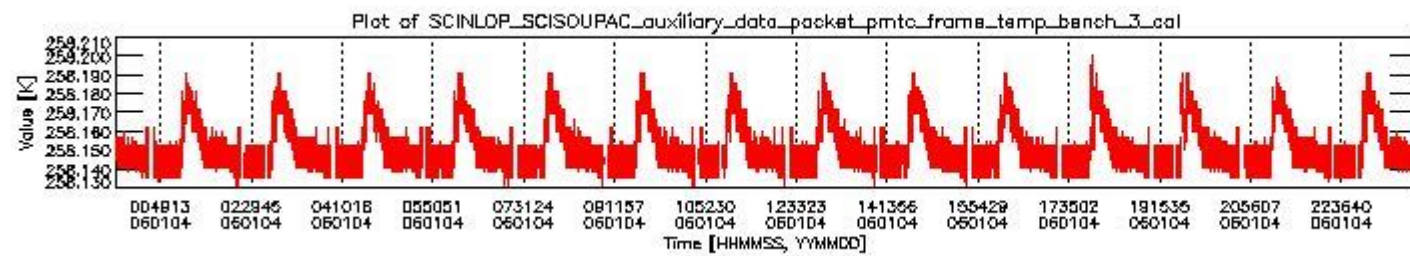
sciamachy_daily_report_level0_PFHS_5_34_N_20060104_2.PNG
