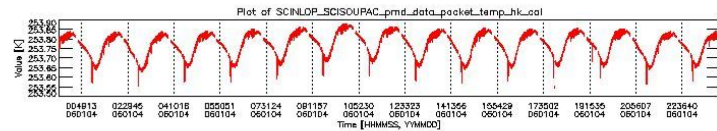
sciamachy_daily_report_level0_PFHS_5_34_N_20060104_3.PNG
