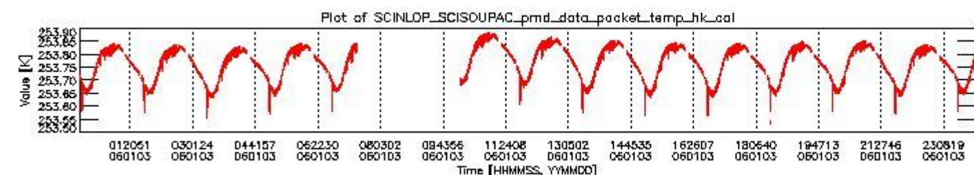
sciamachy_daily_report_level0_PFHS_5_34_N_20060103_3.PNG
