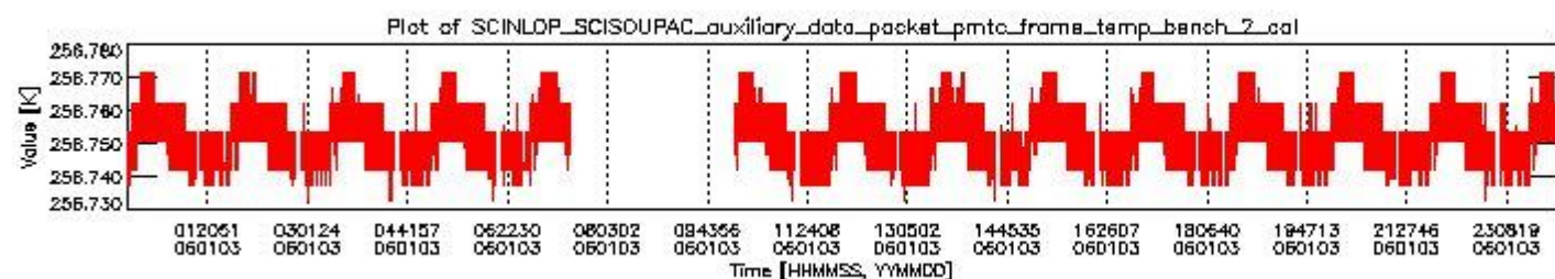
sciamachy_daily_report_level0_PFHS_5_34_N_20060103_1.PNG
