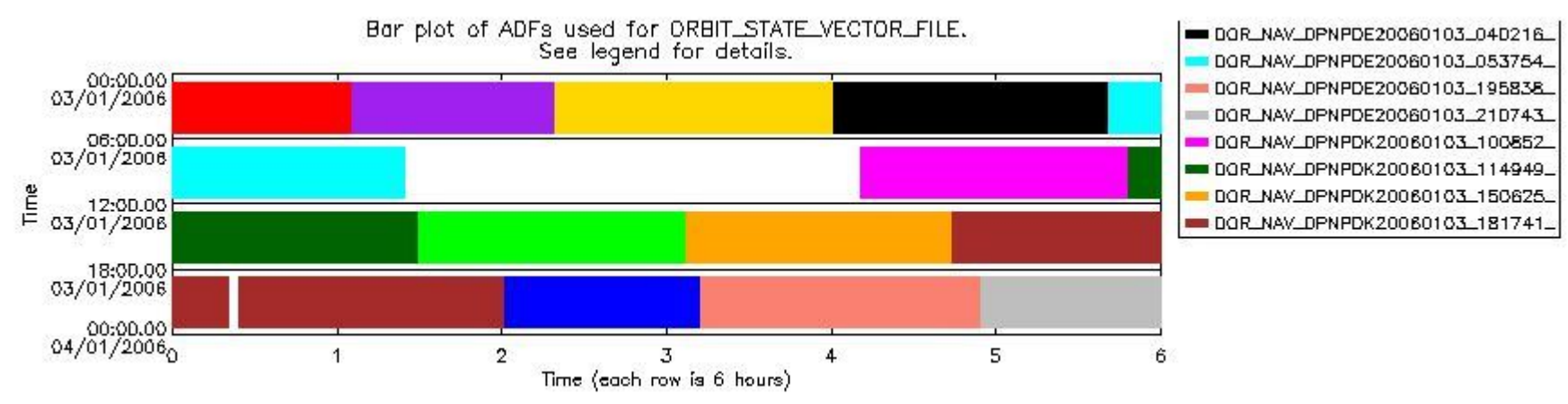
sciamachy_daily_report_level0_PFHS_5_34_N_20060103_6.PNG
