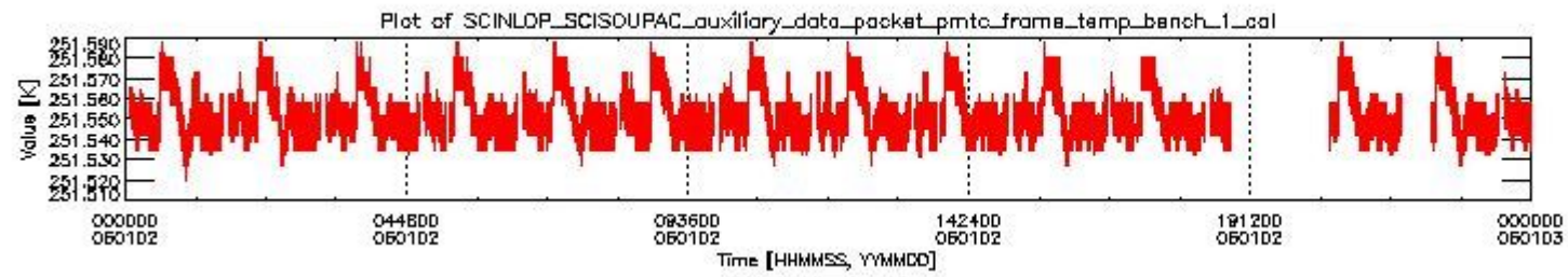
sciamachy_daily_report_level0_PFHS_5_34_N_20060102_0.PNG
