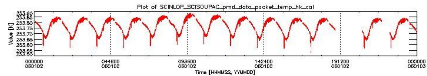
sciamachy_daily_report_level0_PFHS_5_34_N_20060102_3.PNG
