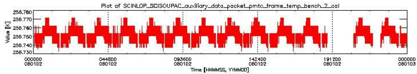
sciamachy_daily_report_level0_PFHS_5_34_N_20060102_1.PNG
