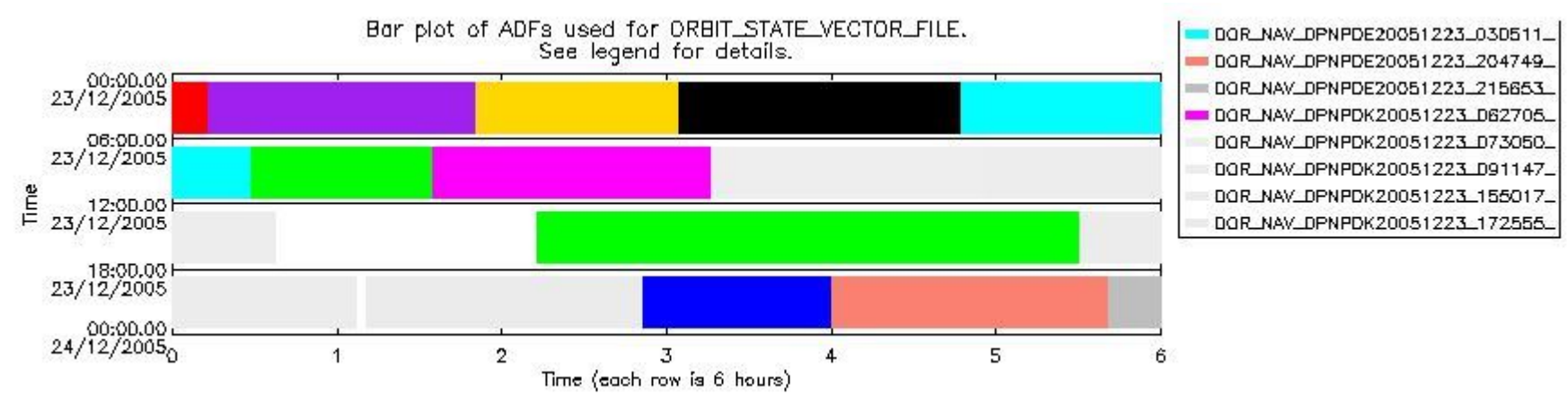
sciamachy_daily_report_level0_PFHS_5_34_N_20051223_6.PNG
