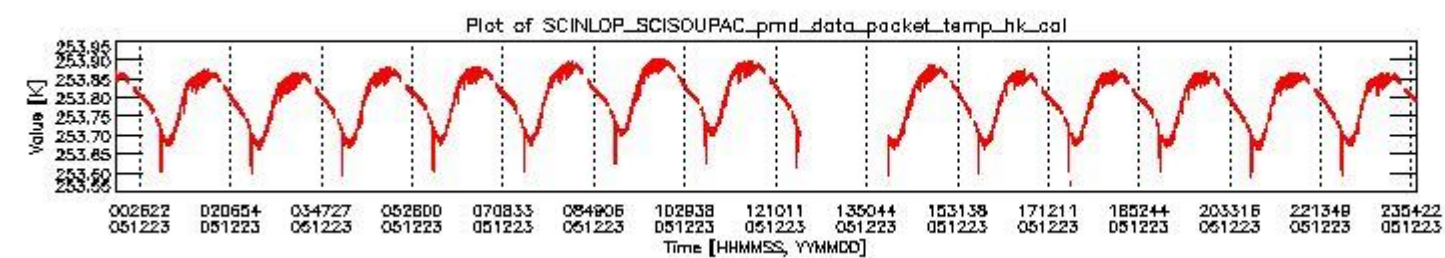
sciamachy_daily_report_level0_PFHS_5_34_N_20051223_3.PNG
