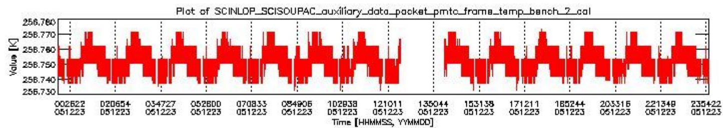
sciamachy_daily_report_level0_PFHS_5_34_N_20051223_1.PNG
