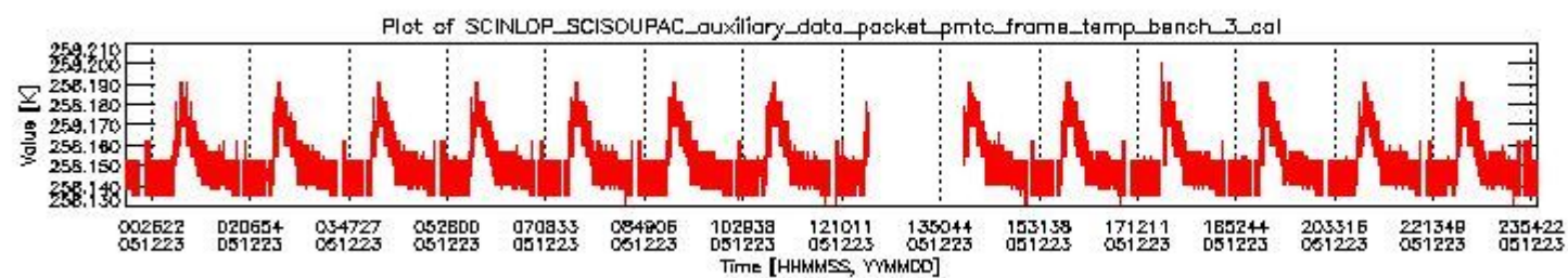
sciamachy_daily_report_level0_PFHS_5_34_N_20051223_2.PNG
