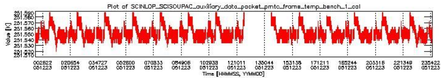
sciamachy_daily_report_level0_PFHS_5_34_N_20051223_0.PNG
