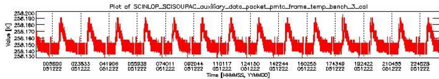
sciamachy_daily_report_level0_PFHS_5_34_N_20051222_2.PNG
