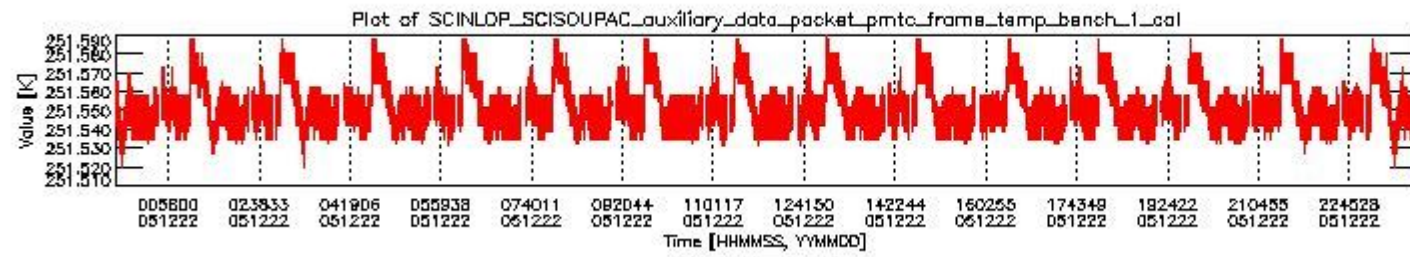
sciamachy_daily_report_level0_PFHS_5_34_N_20051222_0.PNG
