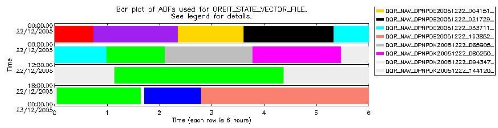
sciamachy_daily_report_level0_PFHS_5_34_N_20051222_6.PNG
