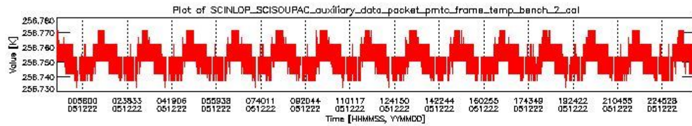
sciamachy_daily_report_level0_PFHS_5_34_N_20051222_1.PNG
