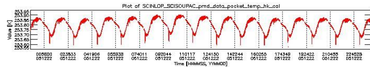
sciamachy_daily_report_level0_PFHS_5_34_N_20051222_3.PNG
