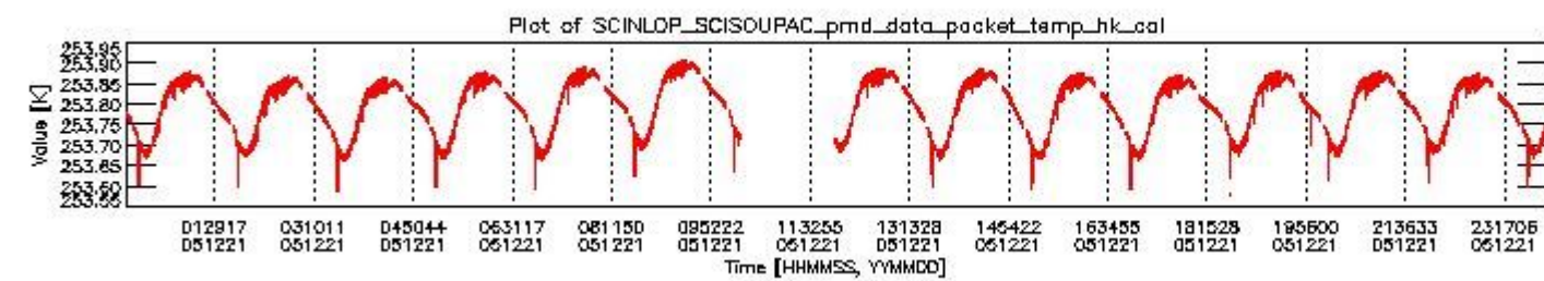
sciamachy_daily_report_level0_PFHS_5_34_N_20051221_3.PNG
