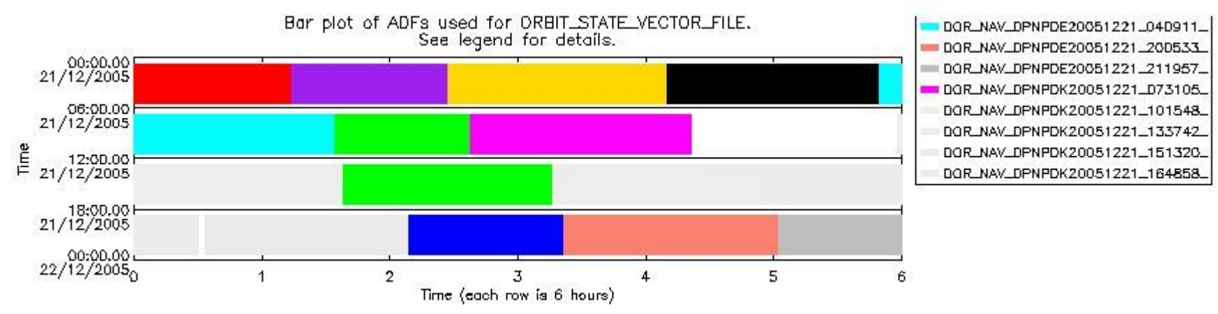
sciamachy_daily_report_level0_PFHS_5_34_N_20051221_6.PNG
