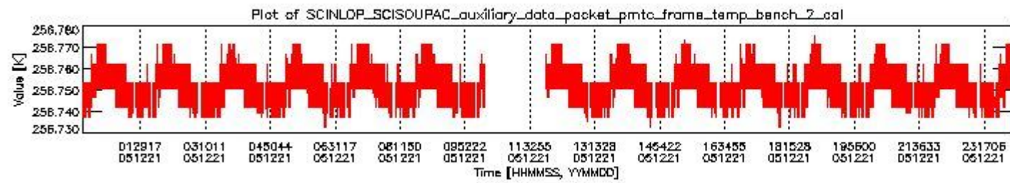
sciamachy_daily_report_level0_PFHS_5_34_N_20051221_1.PNG
