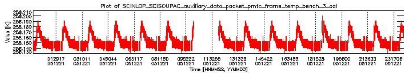
sciamachy_daily_report_level0_PFHS_5_34_N_20051221_2.PNG
