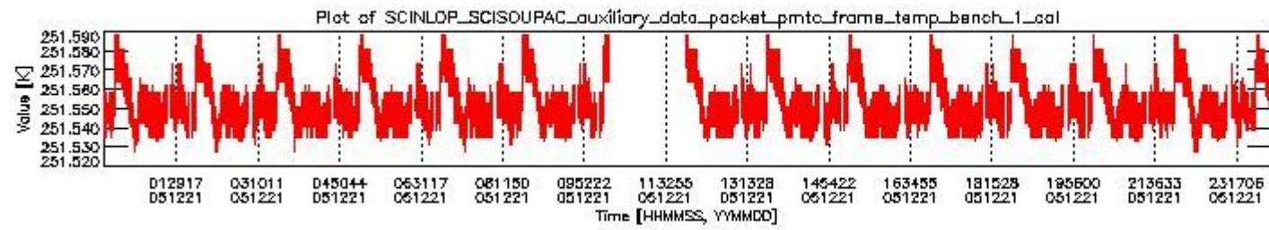
sciamachy_daily_report_level0_PFHS_5_34_N_20051221_0.PNG
