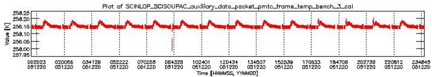
sciamachy_daily_report_level0_PFHS_5_34_N_20051220_2.PNG
