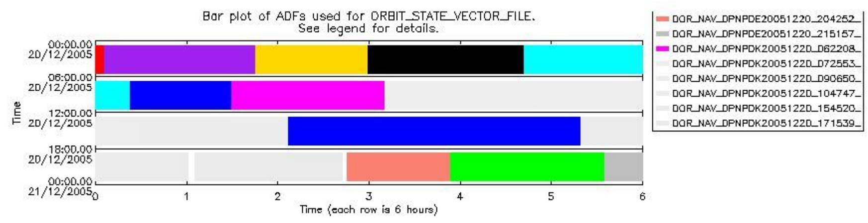
sciamachy_daily_report_level0_PFHS_5_34_N_20051220_6.PNG
