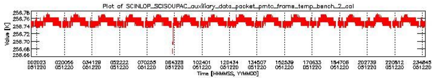
sciamachy_daily_report_level0_PFHS_5_34_N_20051220_1.PNG
