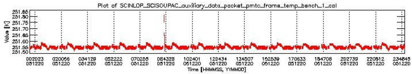
sciamachy_daily_report_level0_PFHS_5_34_N_20051220_0.PNG
