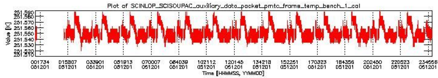
sciamachy_daily_report_level0_PFHS_5_34_N_20051201_0.PNG
