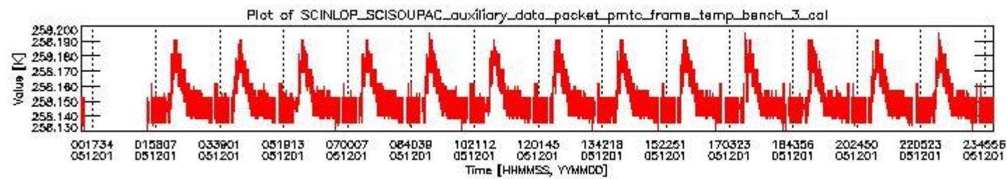
sciamachy_daily_report_level0_PFHS_5_34_N_20051201_2.PNG
