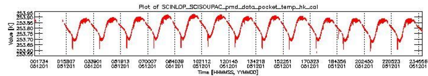
sciamachy_daily_report_level0_PFHS_5_34_N_20051201_3.PNG
