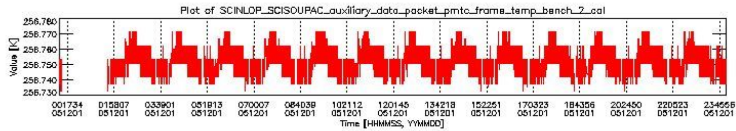
sciamachy_daily_report_level0_PFHS_5_34_N_20051201_1.PNG
