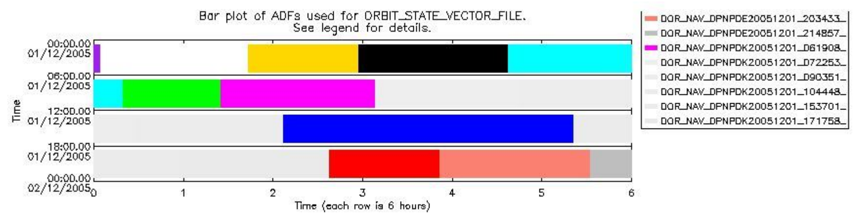
sciamachy_daily_report_level0_PFHS_5_34_N_20051201_6.PNG
