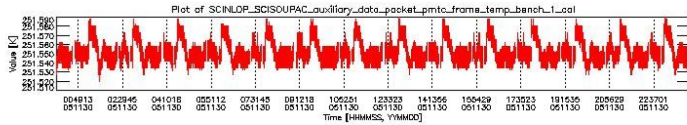
sciamachy_daily_report_level0_PFHS_5_34_N_20051130_0.PNG
