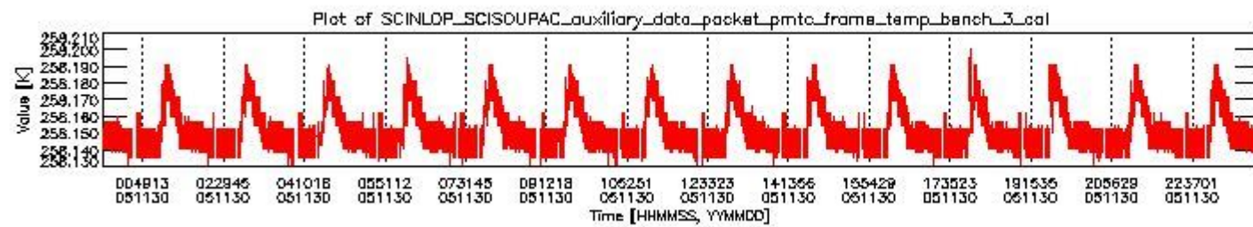
sciamachy_daily_report_level0_PFHS_5_34_N_20051130_2.PNG
