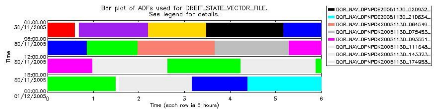
sciamachy_daily_report_level0_PFHS_5_34_N_20051130_6.PNG
