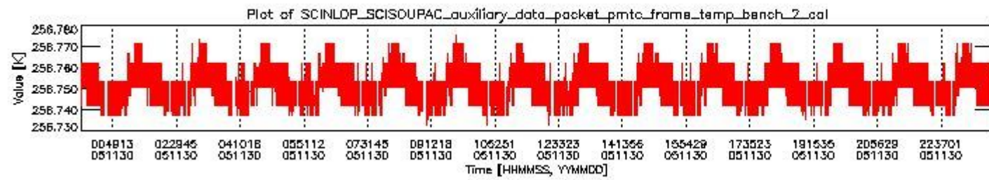
sciamachy_daily_report_level0_PFHS_5_34_N_20051130_1.PNG
