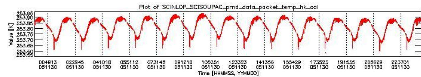
sciamachy_daily_report_level0_PFHS_5_34_N_20051130_3.PNG
