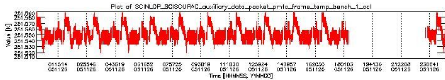
sciamachy_daily_report_level0_PFHS_5_34_N_20051126_0.PNG
