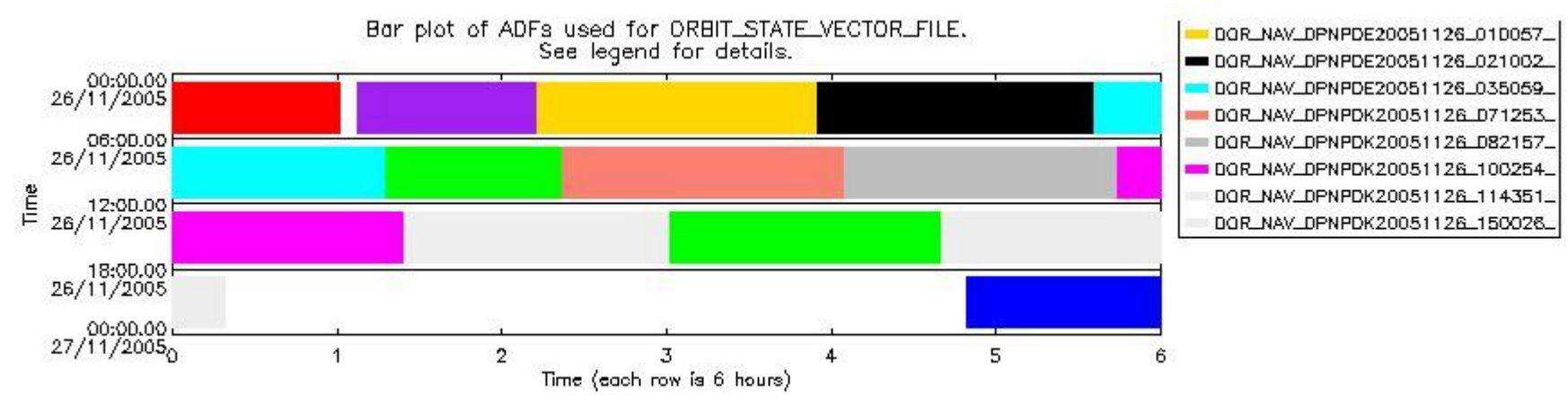
sciamachy_daily_report_level0_PFHS_5_34_N_20051126_6.PNG
