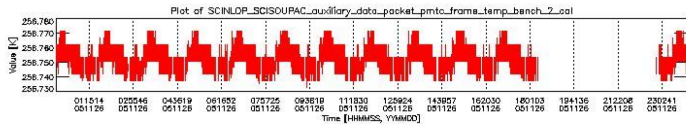
sciamachy_daily_report_level0_PFHS_5_34_N_20051126_1.PNG
