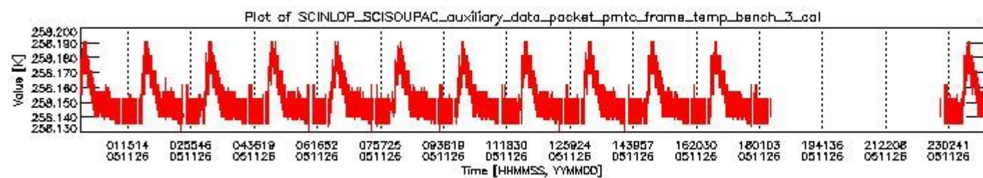
sciamachy_daily_report_level0_PFHS_5_34_N_20051126_2.PNG
