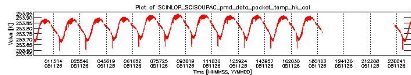
sciamachy_daily_report_level0_PFHS_5_34_N_20051126_3.PNG
