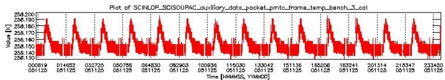
sciamachy_daily_report_level0_PFHS_5_34_N_20051125_2.PNG
