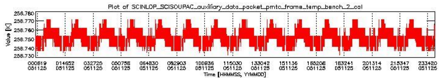
sciamachy_daily_report_level0_PFHS_5_34_N_20051125_1.PNG
