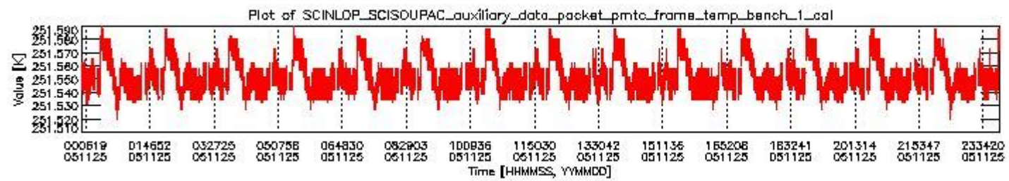
sciamachy_daily_report_level0_PFHS_5_34_N_20051125_0.PNG
