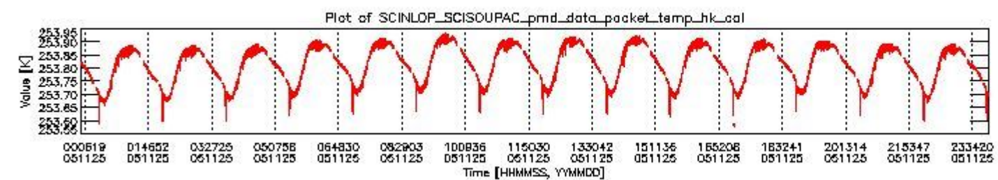
sciamachy_daily_report_level0_PFHS_5_34_N_20051125_3.PNG
