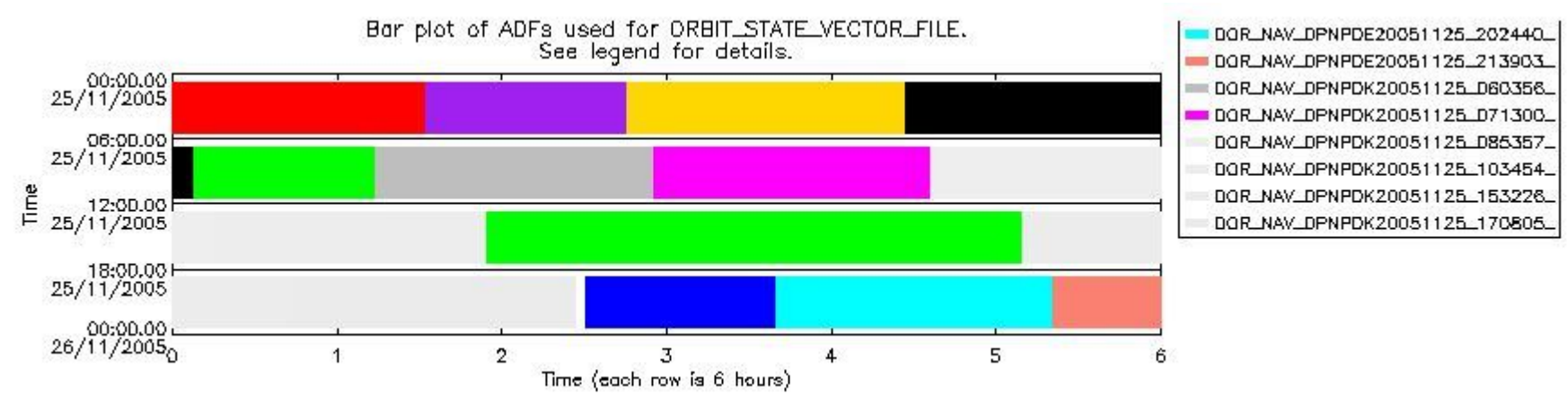
sciamachy_daily_report_level0_PFHS_5_34_N_20051125_6.PNG
