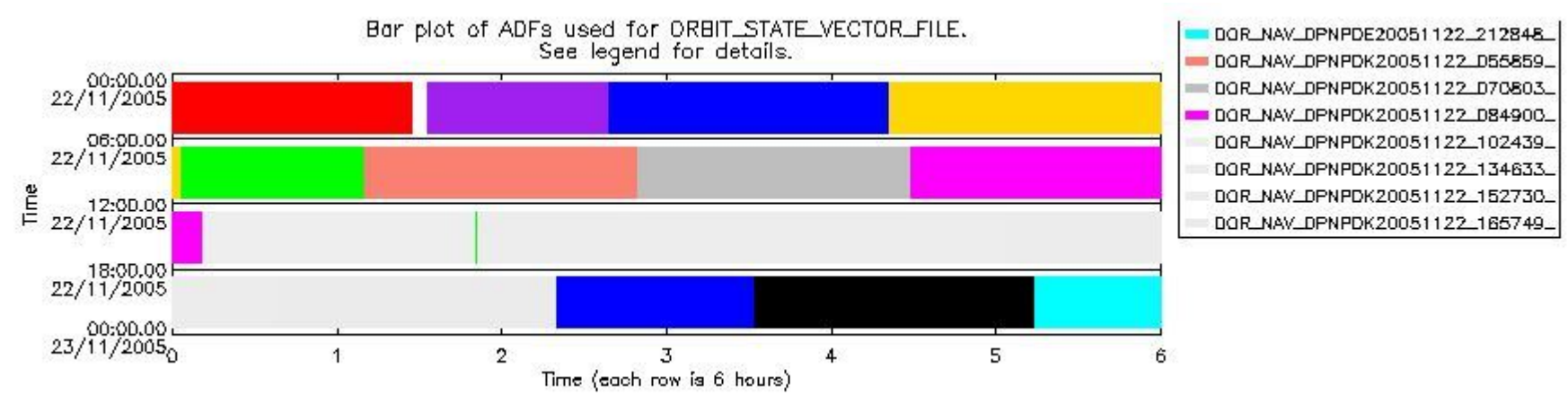
sciamachy_daily_report_level0_PFHS_5_34_N_20051122_6.PNG
