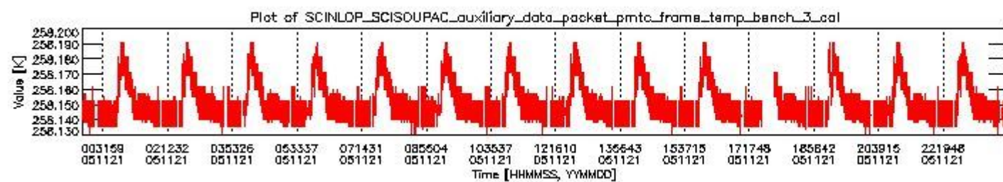
sciamachy_daily_report_level0_PFHS_5_34_N_20051121_2.PNG
