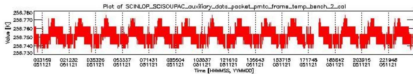
sciamachy_daily_report_level0_PFHS_5_34_N_20051121_1.PNG
