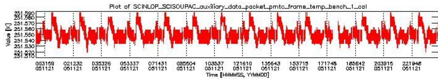
sciamachy_daily_report_level0_PFHS_5_34_N_20051121_0.PNG
