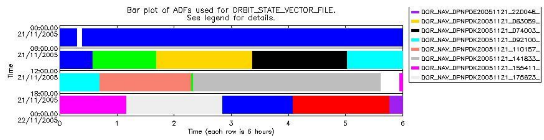
sciamachy_daily_report_level0_PFHS_5_34_N_20051121_6.PNG
