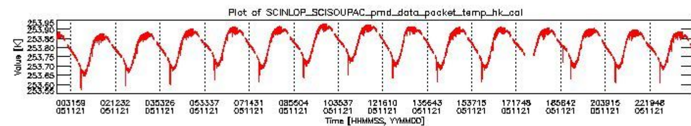
sciamachy_daily_report_level0_PFHS_5_34_N_20051121_3.PNG
