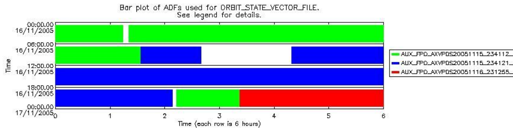
sciamachy_daily_report_level0_PFHS_5_34_N_20051116_6.PNG
