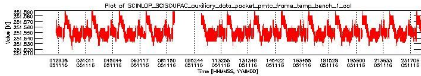
sciamachy_daily_report_level0_PFHS_5_34_N_20051116_0.PNG
