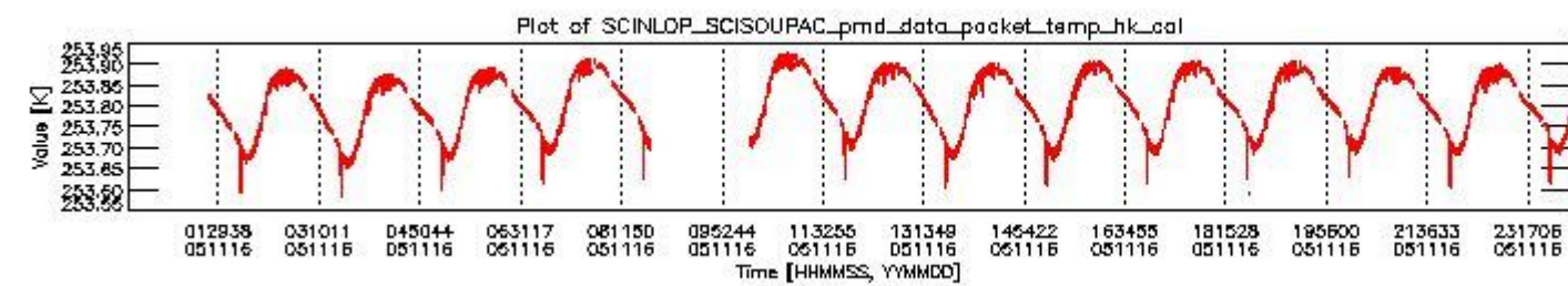
sciamachy_daily_report_level0_PFHS_5_34_N_20051116_3.PNG
