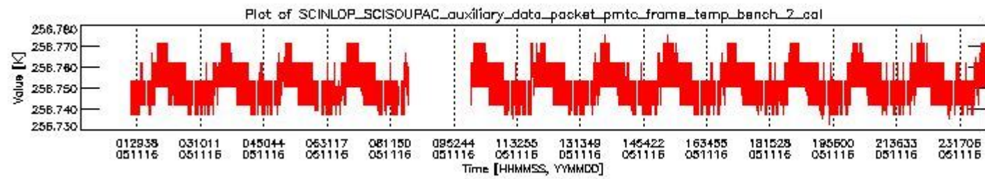
sciamachy_daily_report_level0_PFHS_5_34_N_20051116_1.PNG
