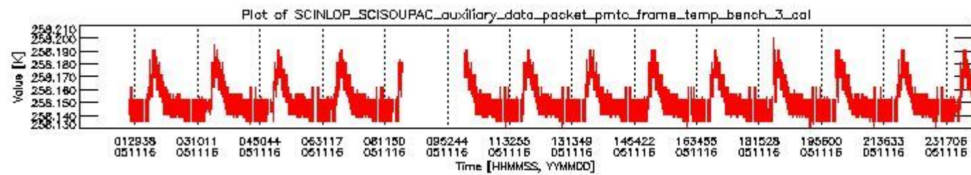
sciamachy_daily_report_level0_PFHS_5_34_N_20051116_2.PNG
