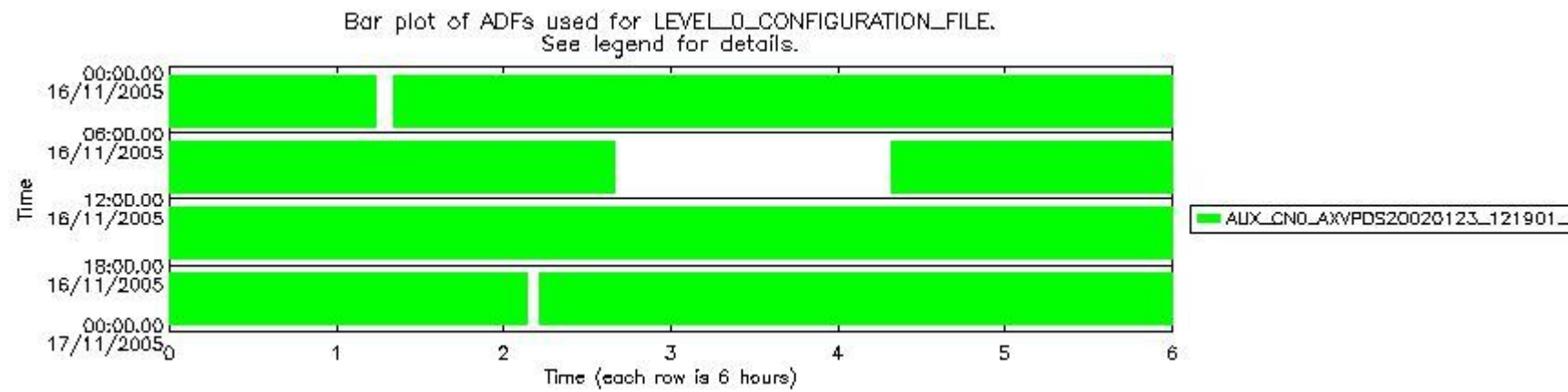
sciamachy_daily_report_level0_PFHS_5_34_N_20051116_5.PNG
