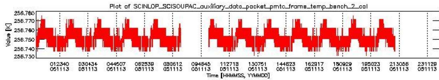
sciamachy_daily_report_level0_PFHS_5_34_N_20051113_1.PNG
