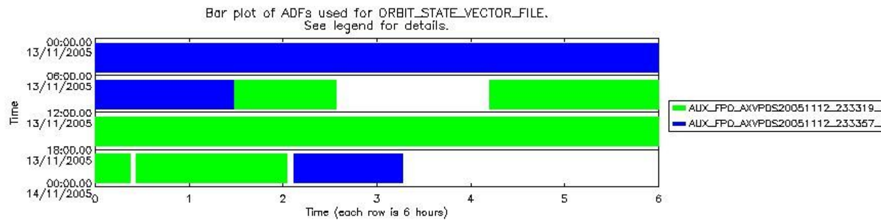
sciamachy_daily_report_level0_PFHS_5_34_N_20051113_6.PNG
