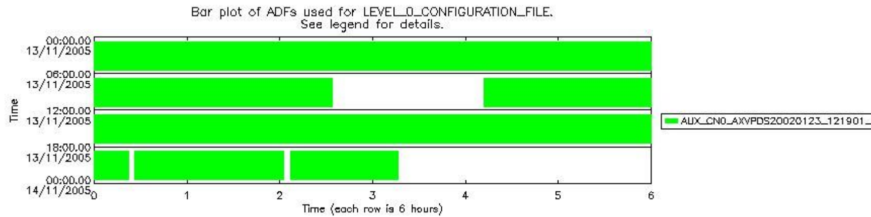
sciamachy_daily_report_level0_PFHS_5_34_N_20051113_5.PNG
