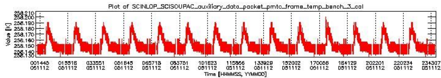
sciamachy_daily_report_level0_PFHS_5_34_N_20051112_2.PNG
