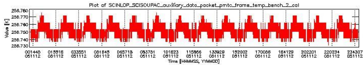
sciamachy_daily_report_level0_PFHS_5_34_N_20051112_1.PNG
