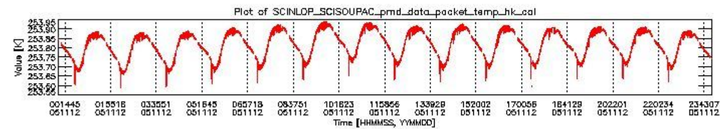
sciamachy_daily_report_level0_PFHS_5_34_N_20051112_3.PNG
