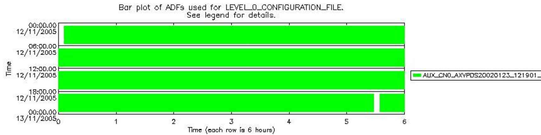
sciamachy_daily_report_level0_PFHS_5_34_N_20051112_5.PNG
