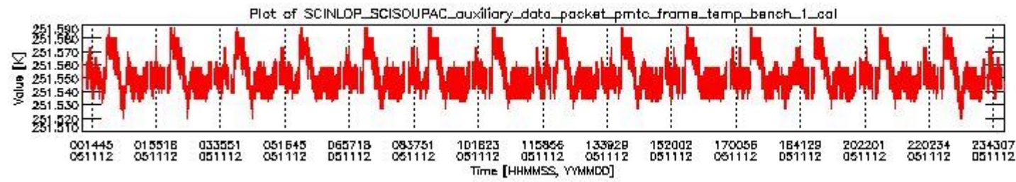
sciamachy_daily_report_level0_PFHS_5_34_N_20051112_0.PNG
