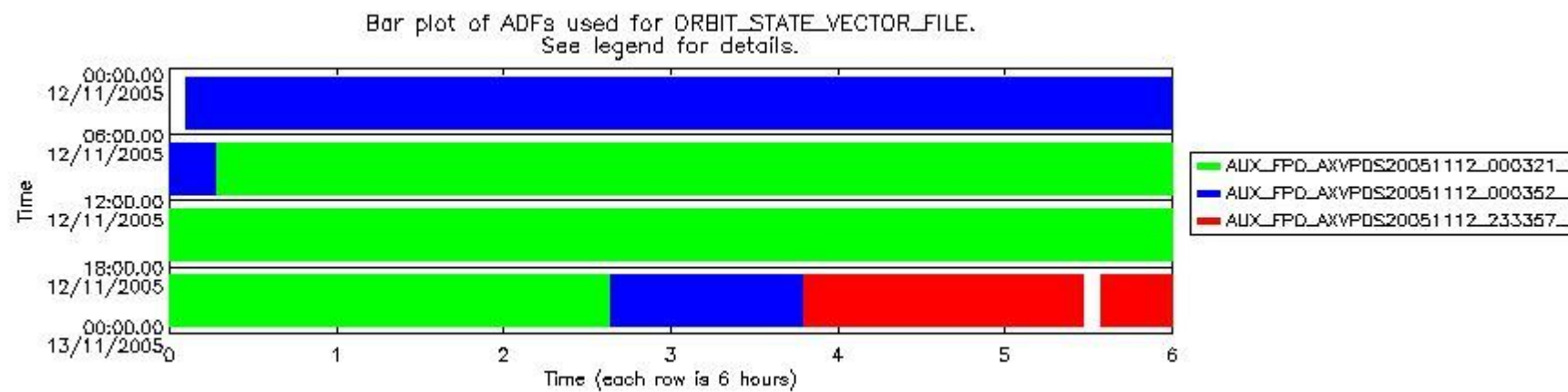
sciamachy_daily_report_level0_PFHS_5_34_N_20051112_6.PNG
