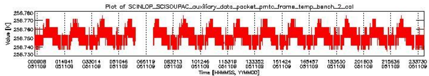
sciamachy_daily_report_level0_PFHS_5_34_N_20051109_1.PNG
