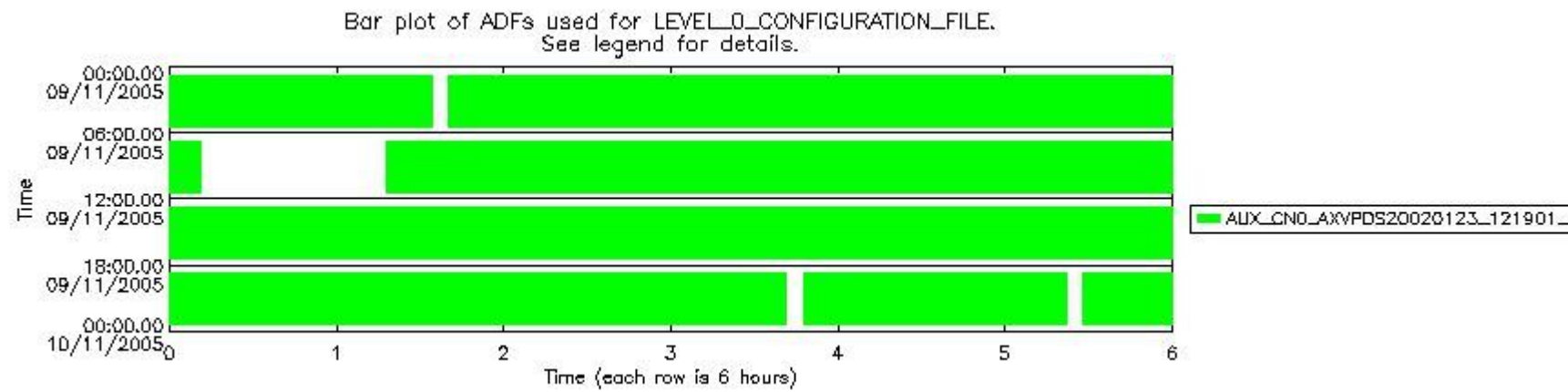
sciamachy_daily_report_level0_PFHS_5_34_N_20051109_5.PNG
