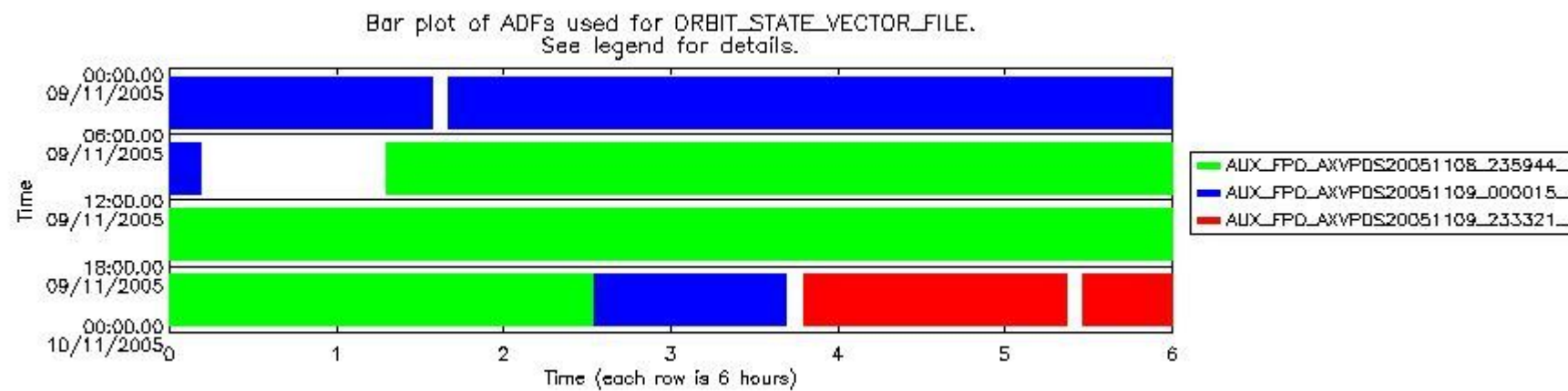
sciamachy_daily_report_level0_PFHS_5_34_N_20051109_6.PNG
