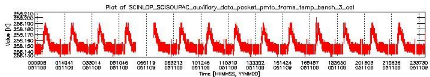
sciamachy_daily_report_level0_PFHS_5_34_N_20051109_2.PNG
