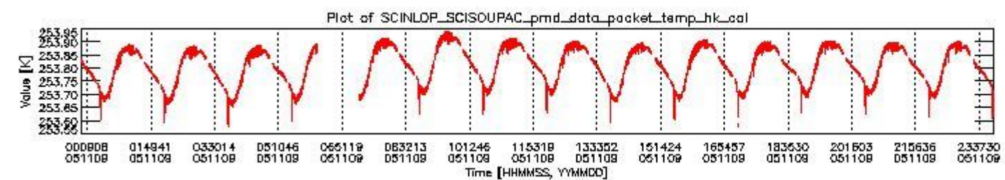
sciamachy_daily_report_level0_PFHS_5_34_N_20051109_3.PNG
