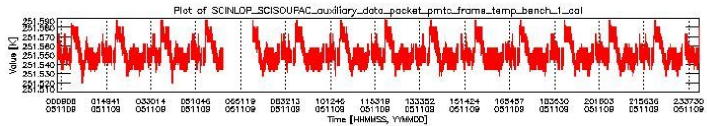
sciamachy_daily_report_level0_PFHS_5_34_N_20051109_0.PNG
