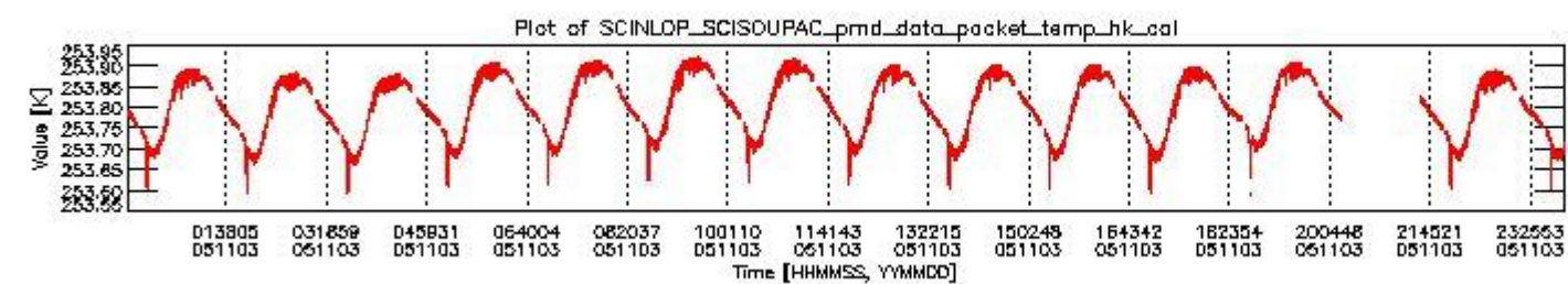
sciamachy_daily_report_level0_PFHS_5_34_N_20051103_3.PNG
