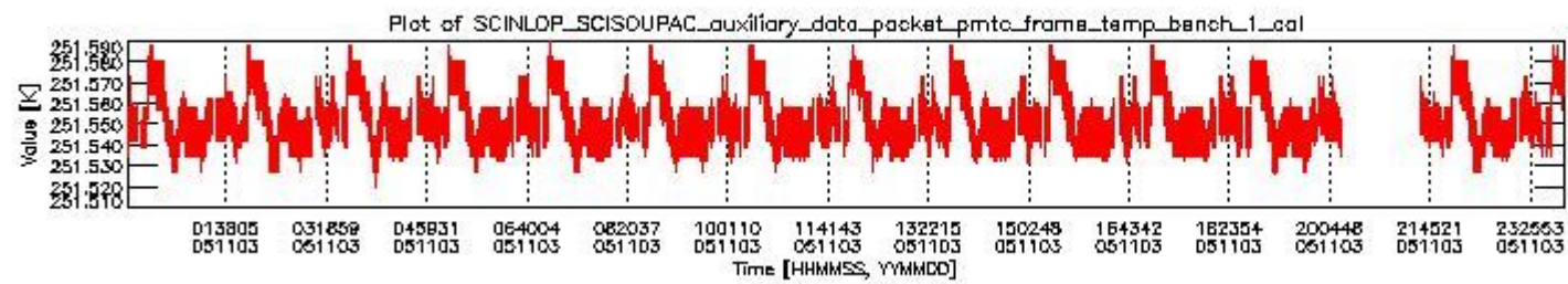
sciamachy_daily_report_level0_PFHS_5_34_N_20051103_0.PNG
