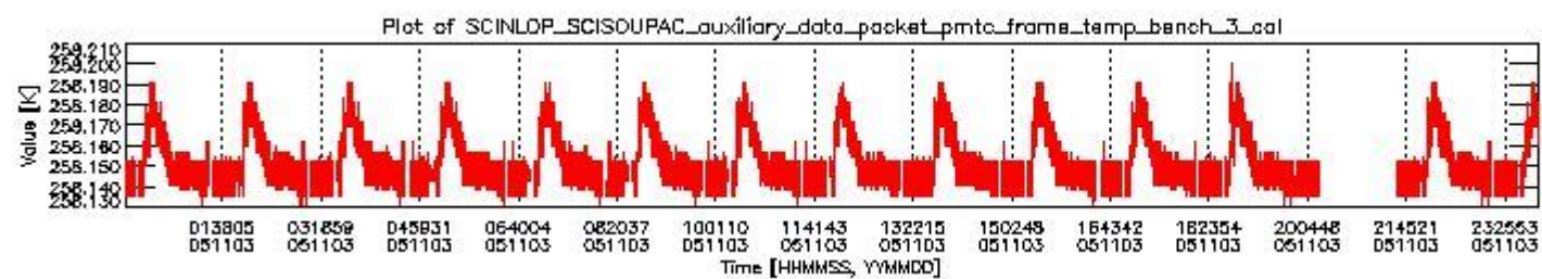
sciamachy_daily_report_level0_PFHS_5_34_N_20051103_2.PNG
