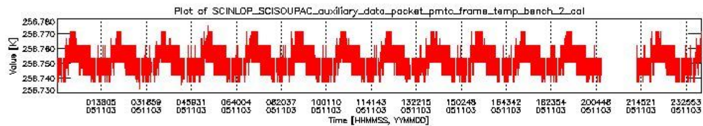
sciamachy_daily_report_level0_PFHS_5_34_N_20051103_1.PNG
