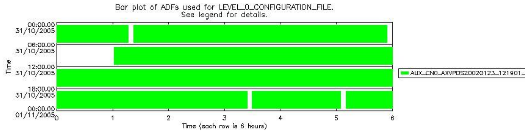
sciamachy_daily_report_level0_PFHS_5_34_N_20051031_5.PNG
