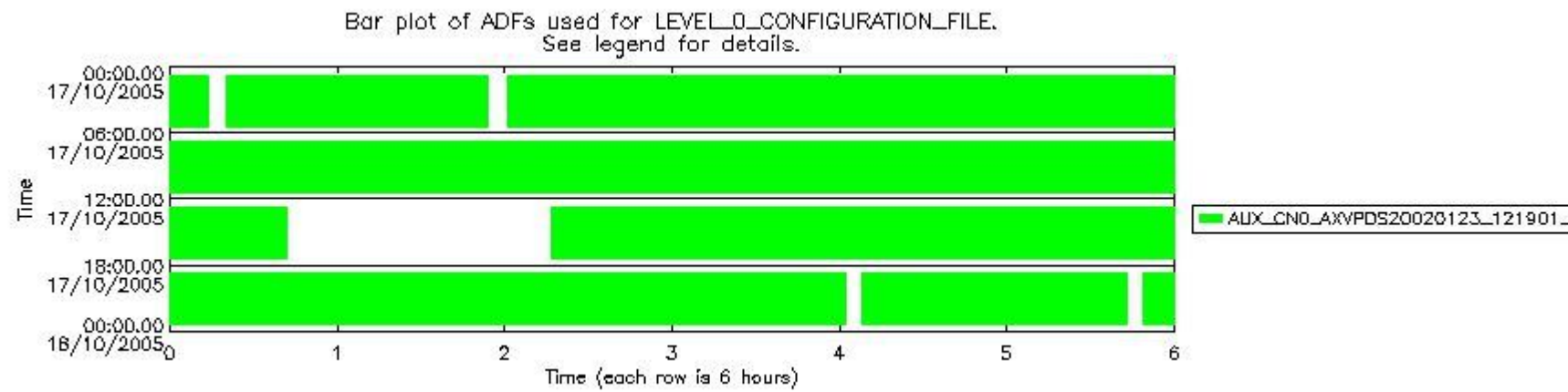
sciamachy_daily_report_level0_PPHS_5_34_N_20051017_5.PNG
