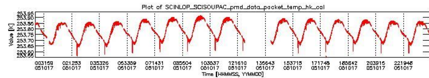
sciamachy_daily_report_level0_PFHS_5_34_N_20051017_3.PNG
