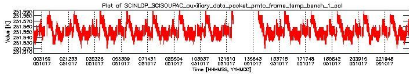
sciamachy_daily_report_level0_PFHS_5_34_N_20051017_0.PNG
