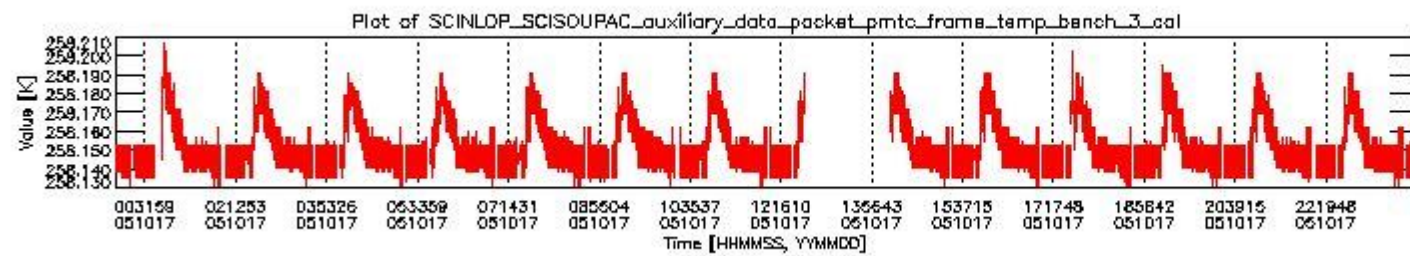
sciamachy_daily_report_level0_PFHS_5_34_N_20051017_2.PNG
