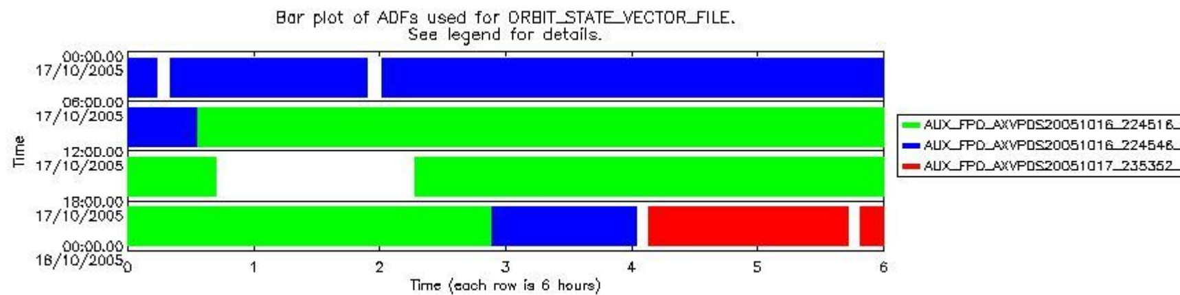
sciamachy_daily_report_level0_PPHS_5_34_N_20051017_6.PNG
