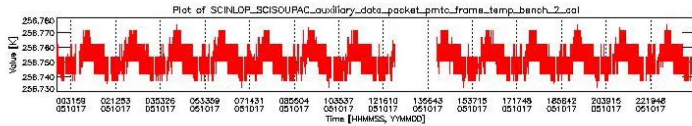
sciamachy_daily_report_level0_PFHS_5_34_N_20051017_1.PNG
