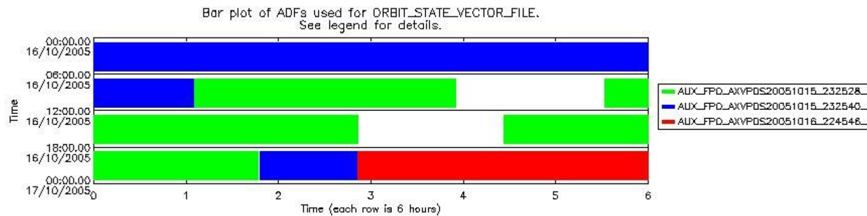
sciamachy_daily_report_level0_PFHS_5_34_N_20051016_6.PNG
