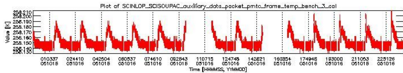
sciamachy_daily_report_level0_PFHS_5_34_N_20051016_2.PNG
