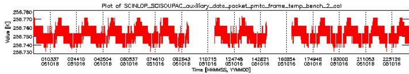
sciamachy_daily_report_level0_PFHS_5_34_N_20051016_1.PNG
