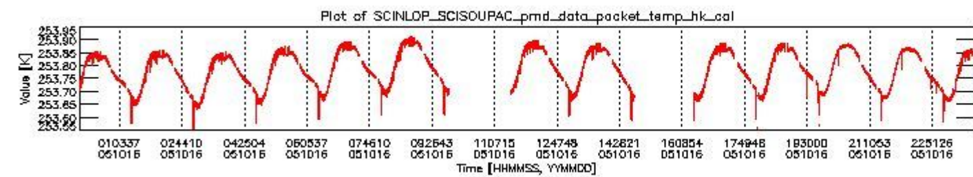
sciamachy_daily_report_level0_PFHS_5_34_N_20051016_3.PNG
