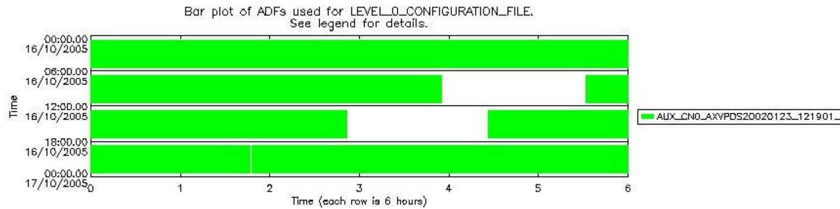
sciamachy_daily_report_level0_PFHS_5_34_N_20051016_5.PNG
