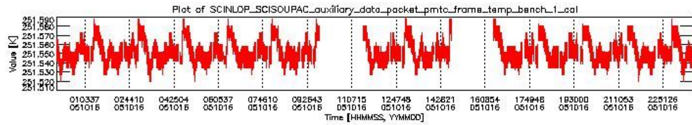
sciamachy_daily_report_level0_PFHS_5_34_N_20051016_0.PNG
