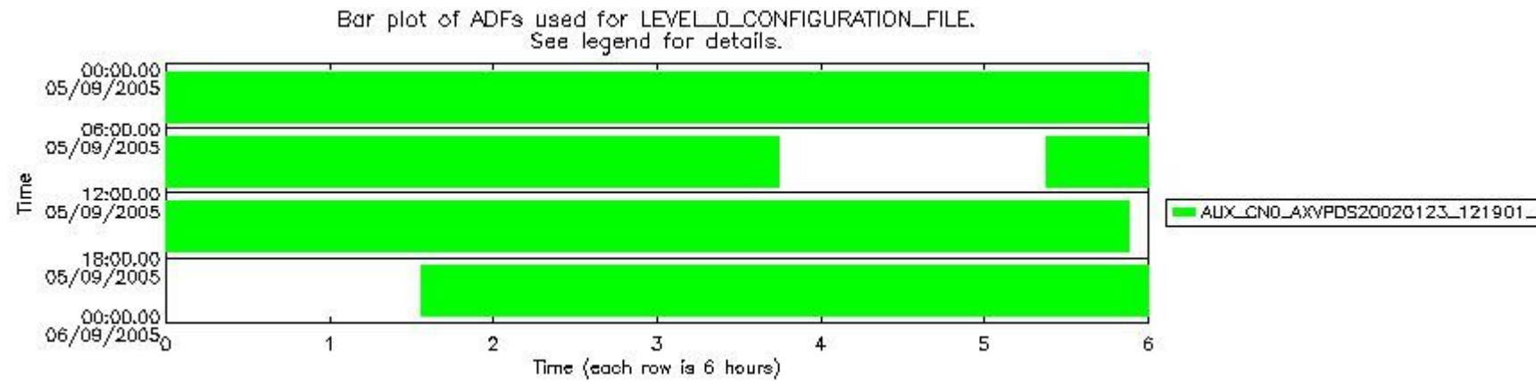
sciamachy_daily_report_level0_PFHS_5_34_N_20050905_5.PNG
