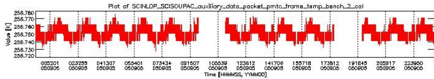
sciamachy_daily_report_level0_PFHS_5_34_N_20050905_1.PNG
