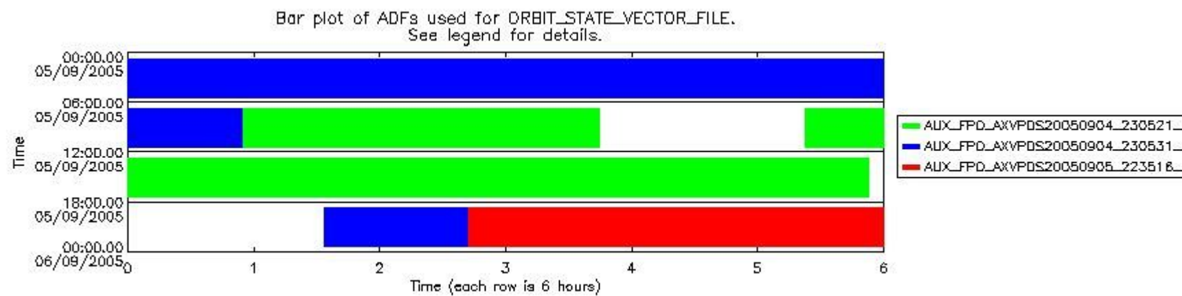
sciamachy_daily_report_level0_PFHS_5_34_N_20050905_6.PNG
