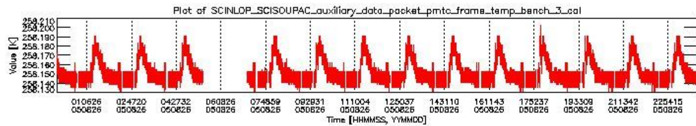
sciamachy_daily_report_level0_PFHS_5_34_N_20050826_2.PNG
