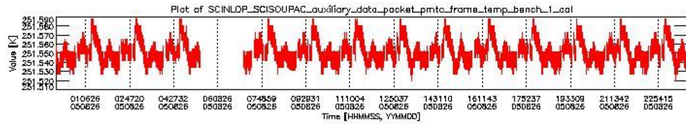
sciamachy_daily_report_level0_PFHS_5_34_N_20050826_0.PNG
