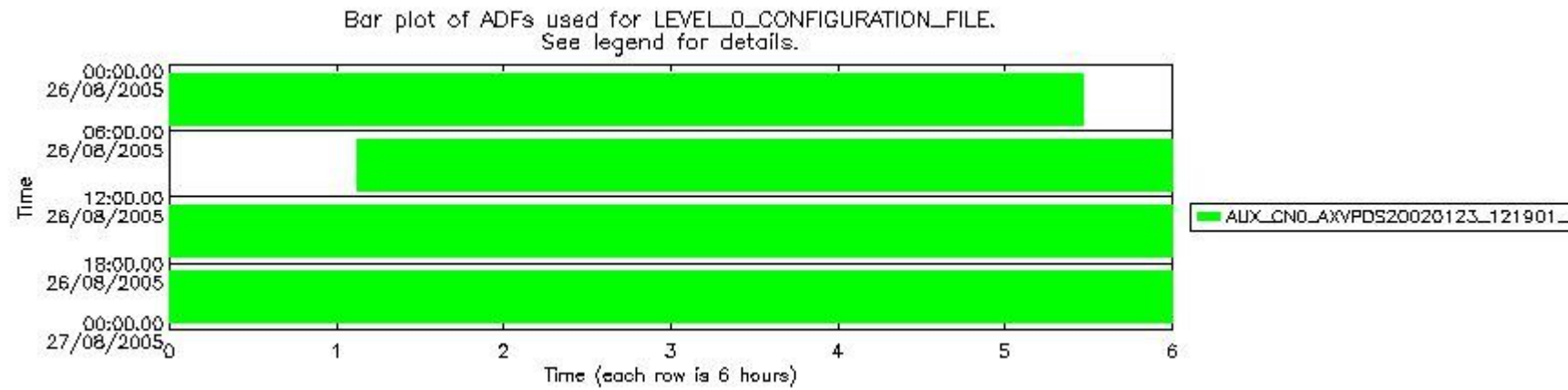
sciamachy_daily_report_level0_PFHS_5_34_N_20050826_5.PNG
