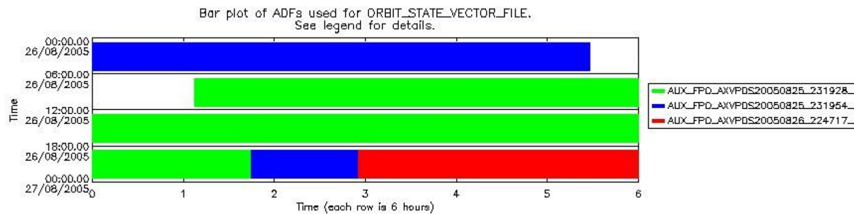
sciamachy_daily_report_level0_PFHS_5_34_N_20050826_6.PNG
