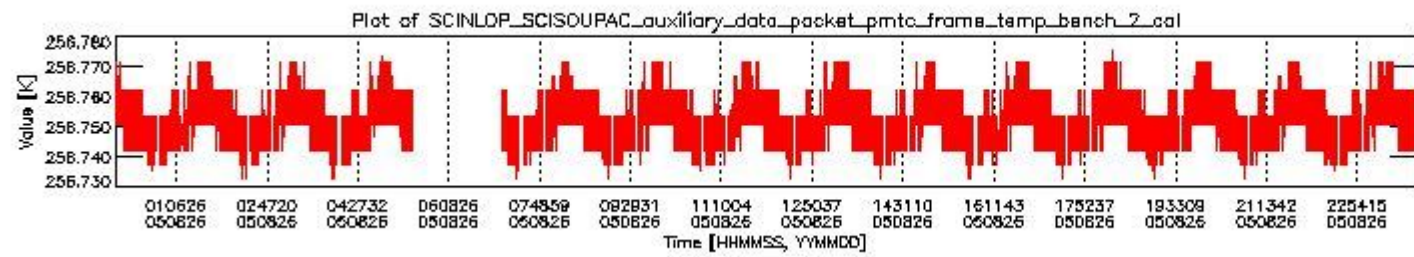
sciamachy_daily_report_level0_PFHS_5_34_N_20050826_1.PNG
