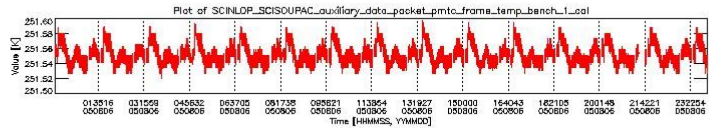
sciamachy_daily_report_level0_PFHS_5_34_N_20050806_0.PNG
