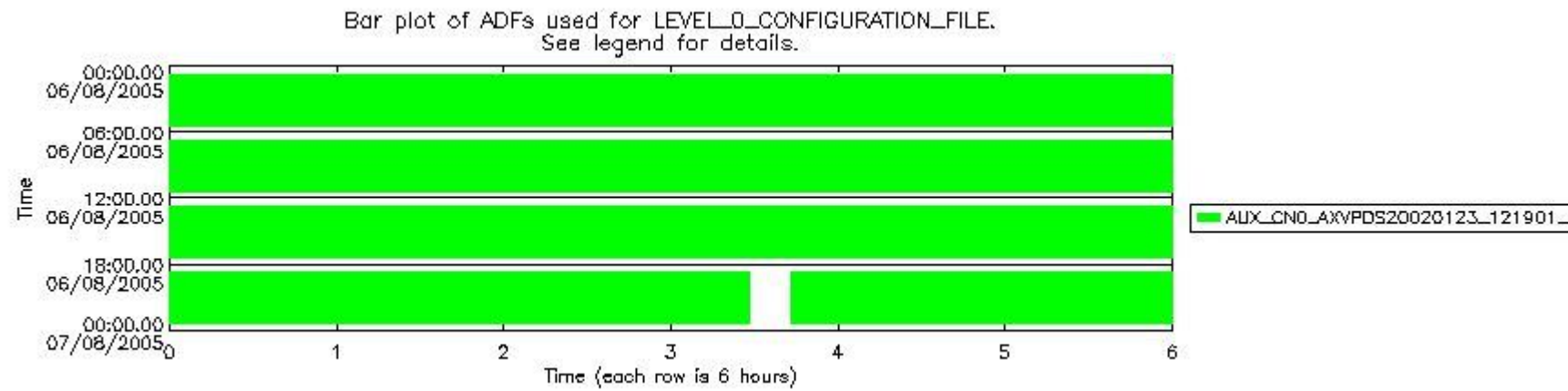
sciamachy_daily_report_level0_PFHS_5_34_N_20050806_5.PNG
