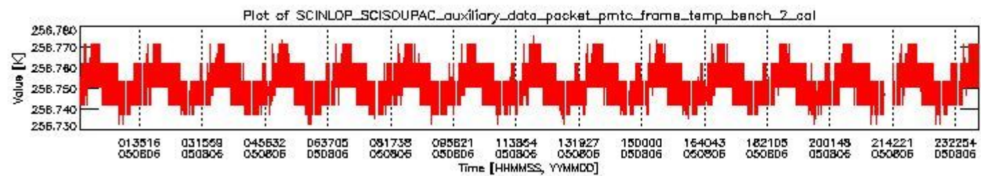
sciamachy_daily_report_level0_PFHS_5_34_N_20050806_1.PNG
