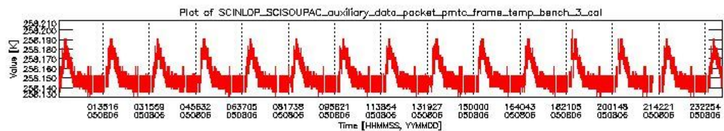
sciamachy_daily_report_level0_PFHS_5_34_N_20050806_2.PNG
