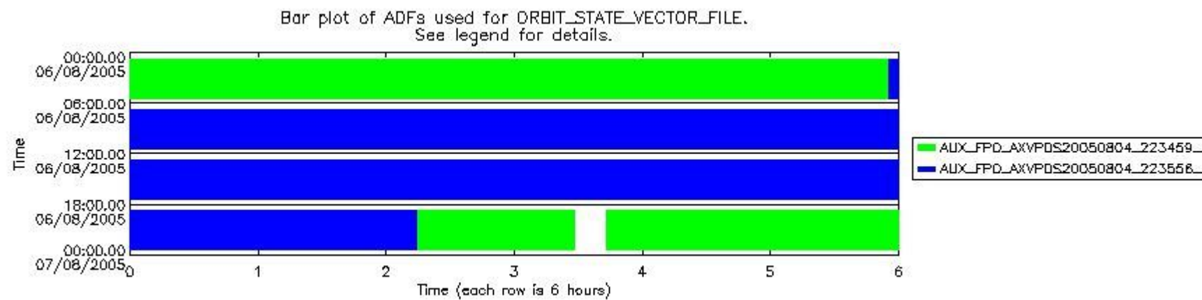
sciamachy_daily_report_level0_PFHS_5_34_N_20050806_6.PNG
