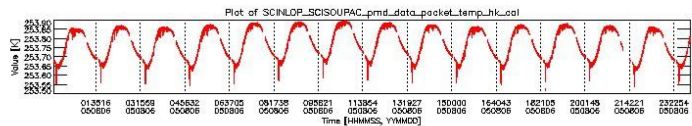
sciamachy_daily_report_level0_PFHS_5_34_N_20050806_3.PNG
