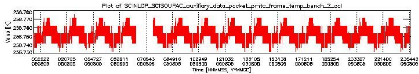
sciamachy_daily_report_level0_PFHS_5_34_N_20050805_1.PNG
