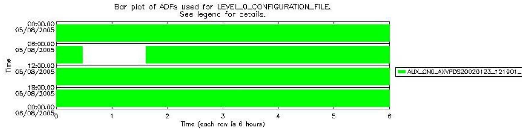
sciamachy_daily_report_level0_PFHS_5_34_N_20050805_5.PNG
