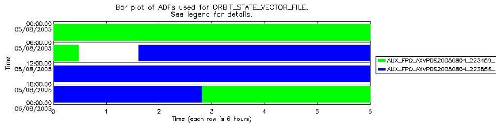
sciamachy_daily_report_level0_PFHS_5_34_N_20050805_6.PNG
