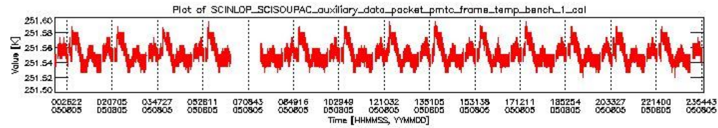
sciamachy_daily_report_level0_PFHS_5_34_N_20050805_0.PNG
