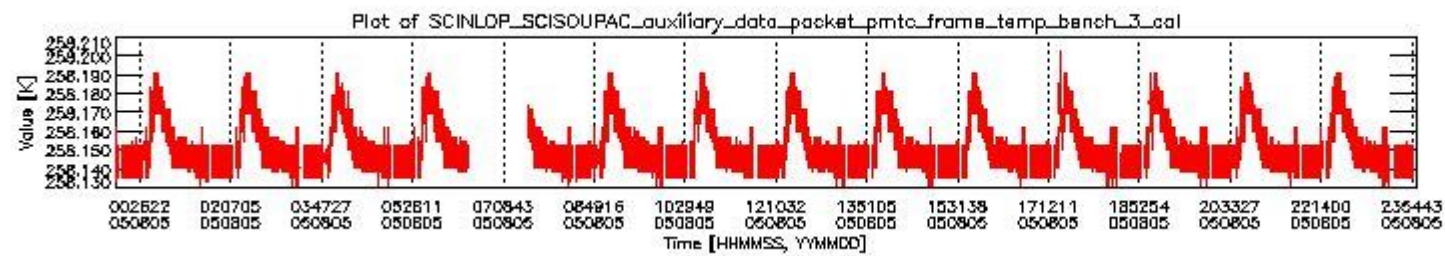
sciamachy_daily_report_level0_PFHS_5_34_N_20050805_2.PNG
