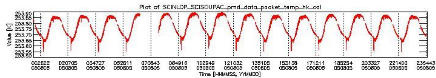
sciamachy_daily_report_level0_PFHS_5_34_N_20050805_3.PNG
