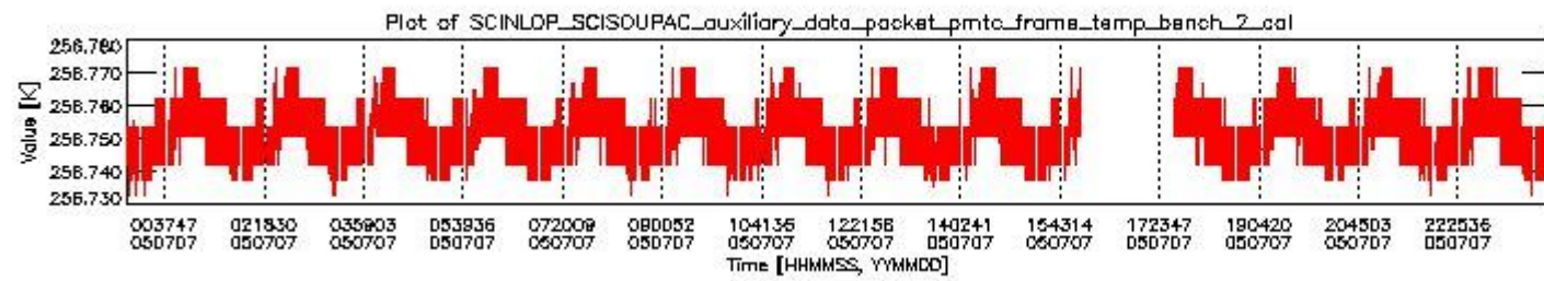
sciamachy_daily_report_level0_PFHS_5_33_N_20050707_1.PNG
