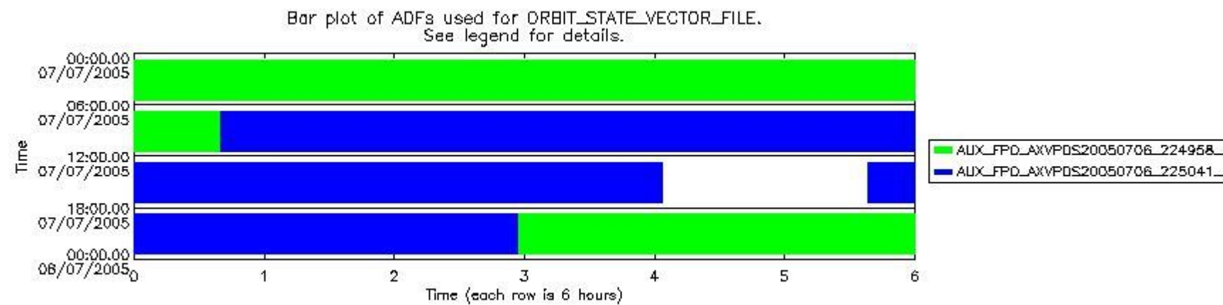
sciamachy_daily_report_level0_PFHS_5_33_N_20050707_6.PNG
