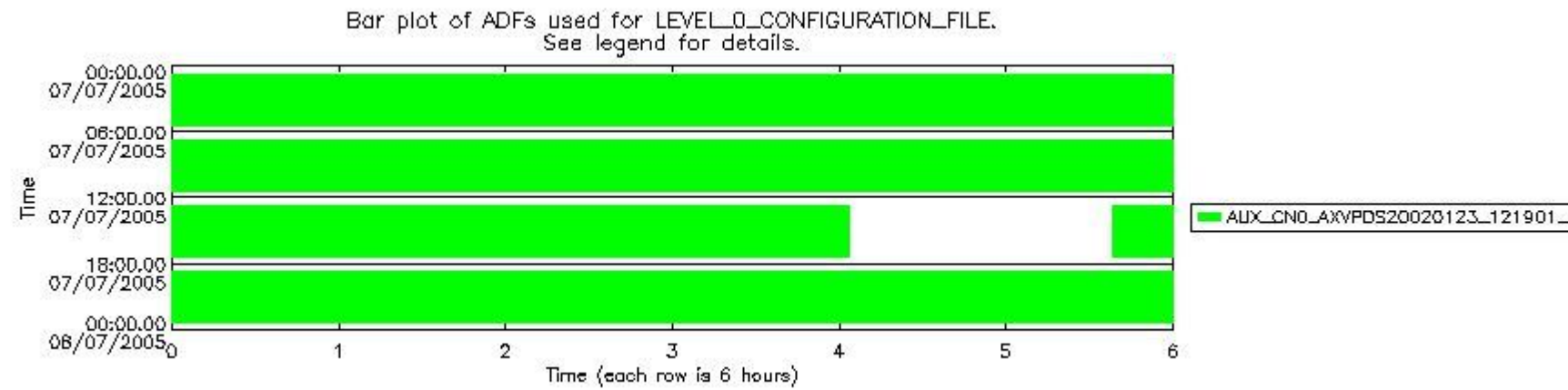
sciamachy_daily_report_level0_PFHS_5_33_N_20050707_5.PNG
