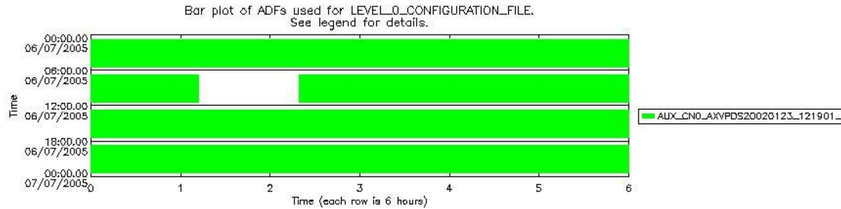
sciamachy_daily_report_level0_PFHS_5_33_N_20050706_5.PNG
