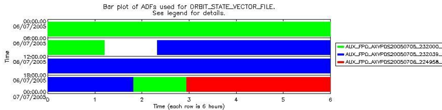
sciamachy_daily_report_level0_PFHS_5_33_N_20050706_6.PNG
