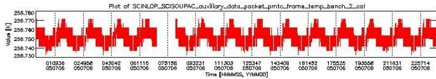
sciamachy_daily_report_level0_PFHS_5_33_N_20050706_1.PNG
