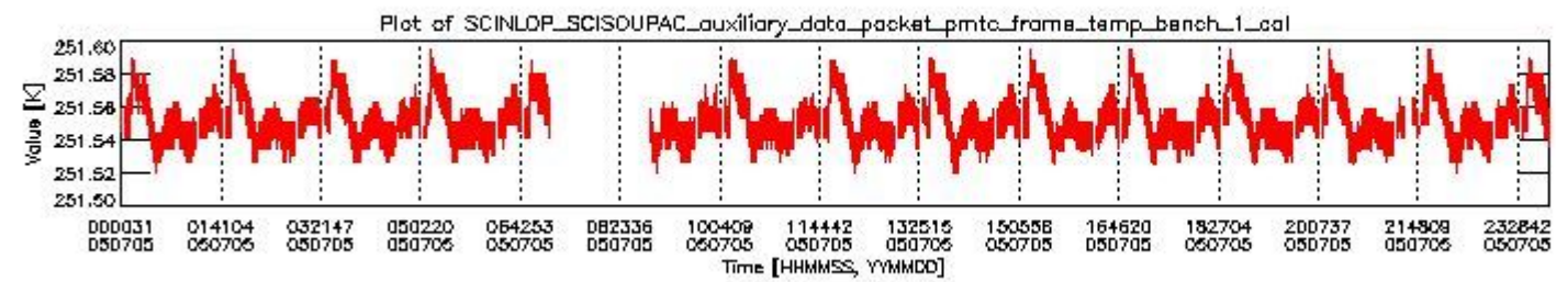
sciamachy_daily_report_level0_PFHS_5_33_N_20050705_0.PNG
