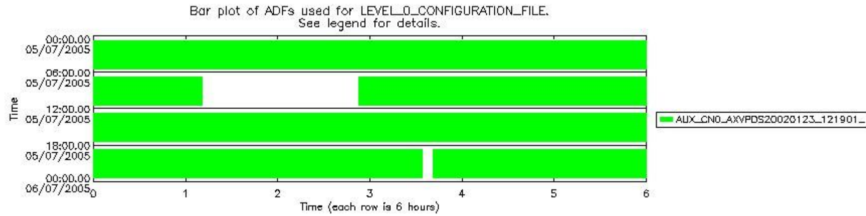
sciamachy_daily_report_level0_PFHS_5_33_N_20050705_5.PNG
