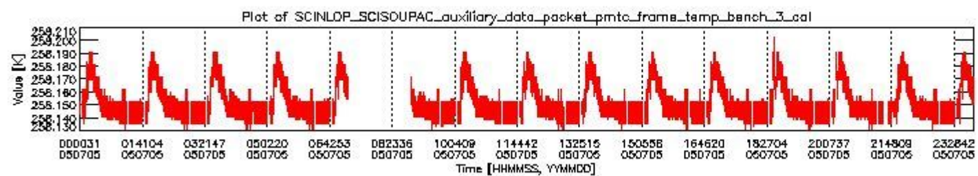
sciamachy_daily_report_level0_PFHS_5_33_N_20050705_2.PNG
