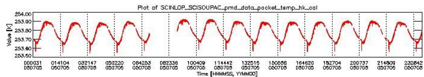
sciamachy_daily_report_level0_PFHS_5_33_N_20050705_3.PNG
