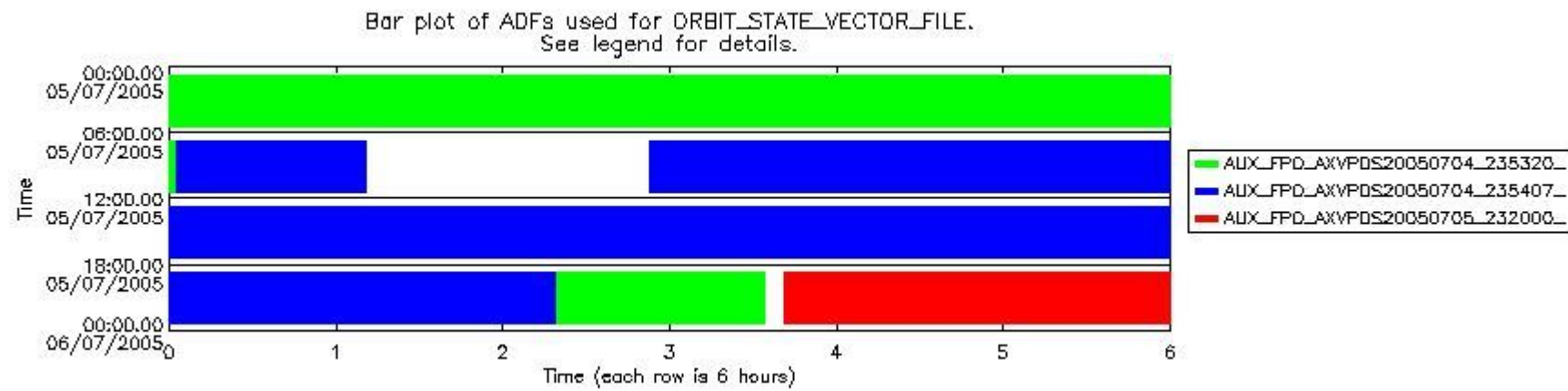
sciamachy_daily_report_level0_PFHS_5_33_N_20050705_6.PNG
