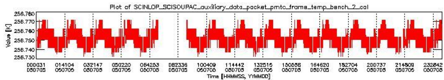
sciamachy_daily_report_level0_PFHS_5_33_N_20050705_1.PNG
