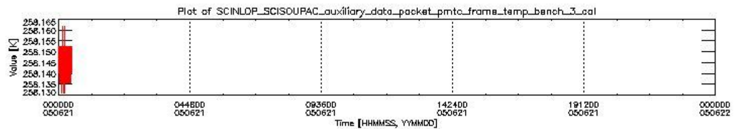
sciamachy_daily_report_level0_PFHS_5_33_N_20050621_2.PNG
