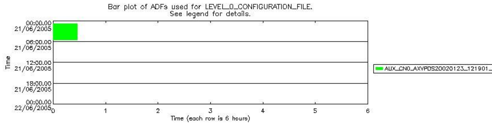
sciamachy_daily_report_level0_PFHS_5_33_N_20050621_5.PNG
