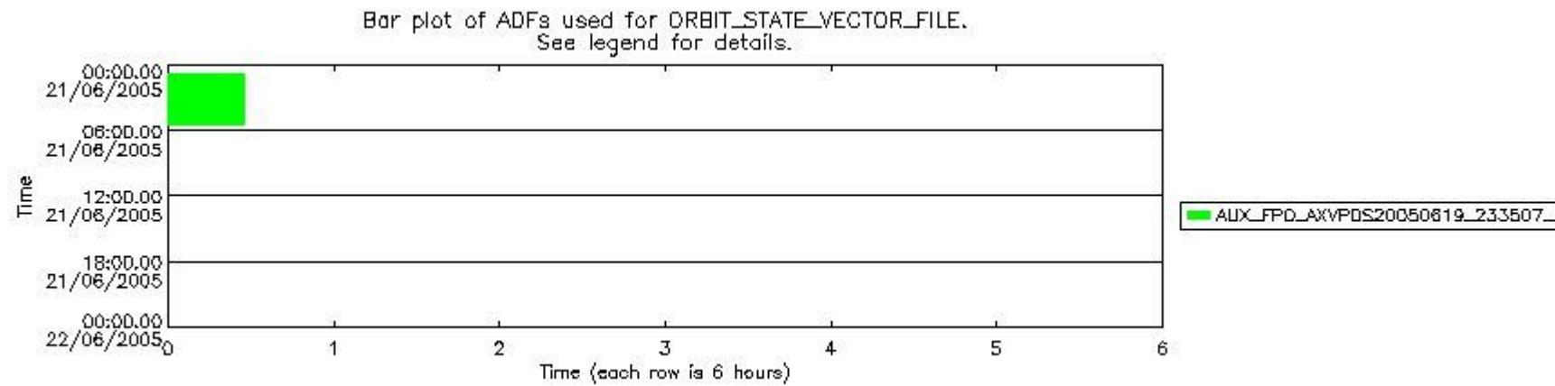
sciamachy_daily_report_level0_PFHS_5_33_N_20050621_6.PNG
