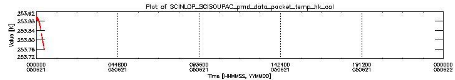
sciamachy_daily_report_level0_PFHS_5_33_N_20050621_3.PNG
