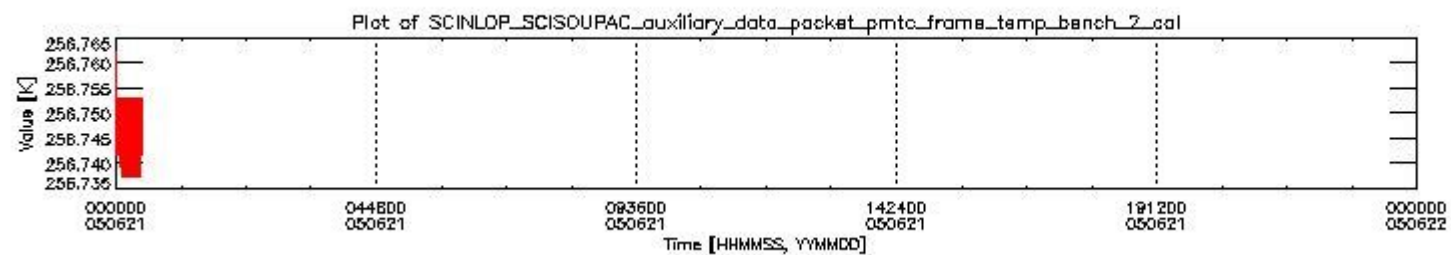
sciamachy_daily_report_level0_PFHS_5_33_N_20050621_0.PNG
