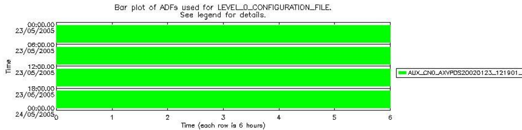
sciamachy_daily_report_level0_PFHS_5_32_N_20050523_5.PNG
