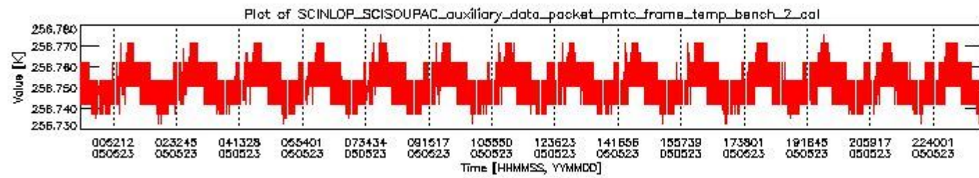
sciamachy_daily_report_level0_PFHS_5_32_N_20050523_1.PNG
