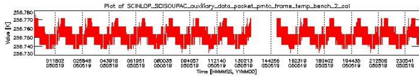
sciamachy_daily_report_level0_PFHS_5_32_N_20050519_1.PNG
