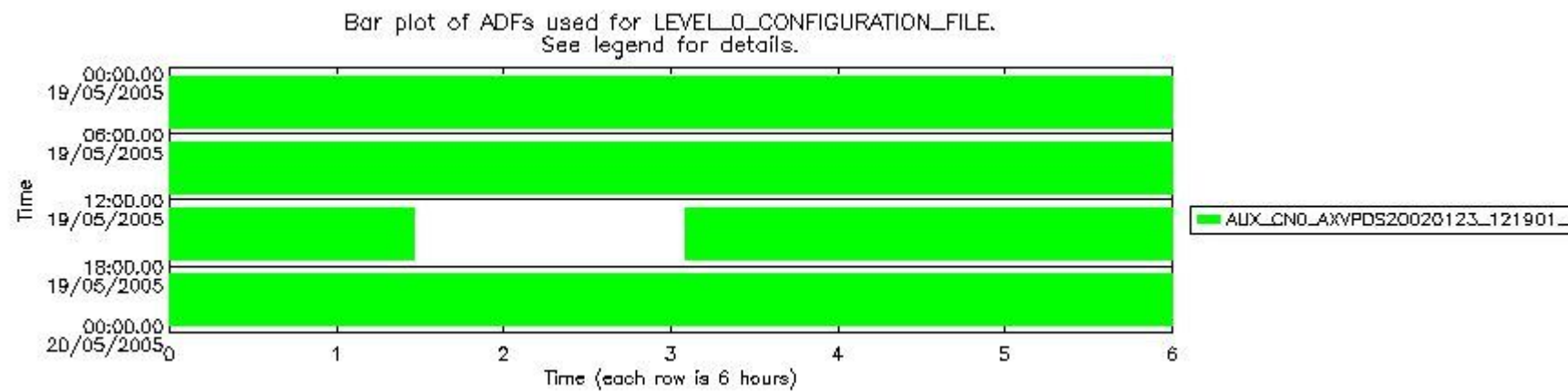
sciamachy_daily_report_level0_PFHS_5_32_N_20050519_5.PNG
