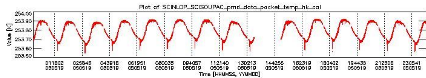
sciamachy_daily_report_level0_PFHS_5_32_N_20050519_3.PNG
