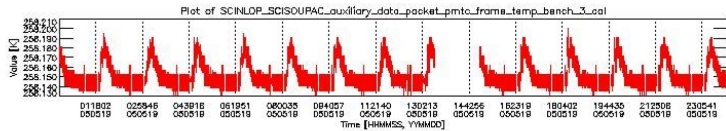
sciamachy_daily_report_level0_PFHS_5_32_N_20050519_2.PNG
