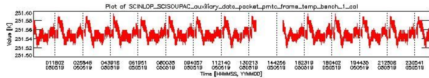
sciamachy_daily_report_level0_PFHS_5_32_N_20050519_0.PNG
