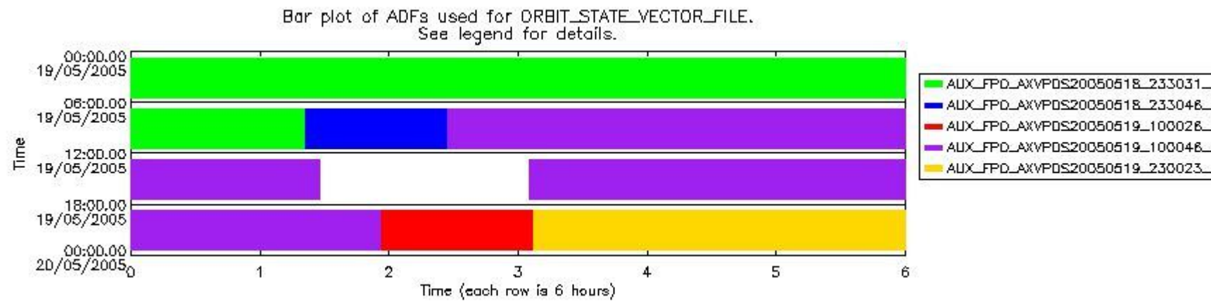
sciamachy_daily_report_level0_PFHS_5_32_N_20050519_6.PNG
