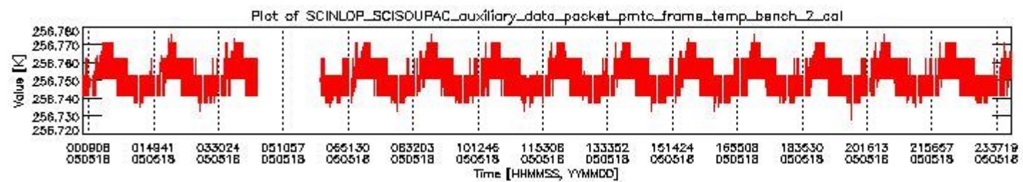
sciamachy_daily_report_level0_PFHS_5_32_N_20050518_1.PNG
