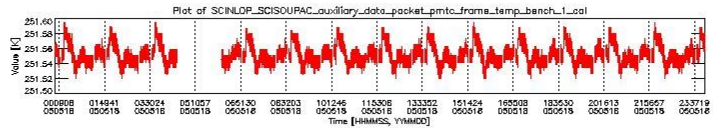
sciamachy_daily_report_level0_PFHS_5_32_N_20050518_0.PNG
