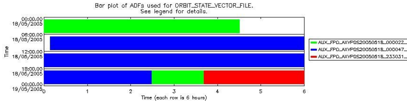
sciamachy_daily_report_level0_PFHS_5_32_N_20050518_6.PNG
