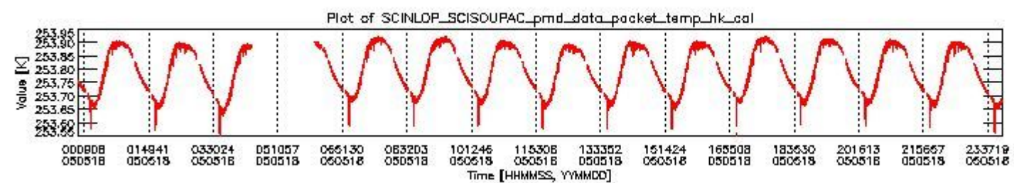
sciamachy_daily_report_level0_PFHS_5_32_N_20050518_3.PNG
