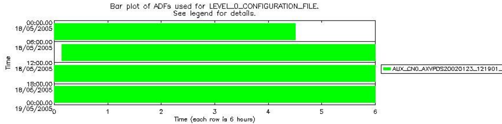
sciamachy_daily_report_level0_PFHS_5_32_N_20050518_5.PNG
