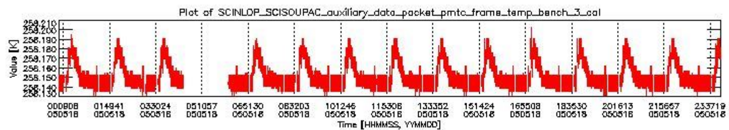
sciamachy_daily_report_level0_PFHS_5_32_N_20050518_2.PNG
