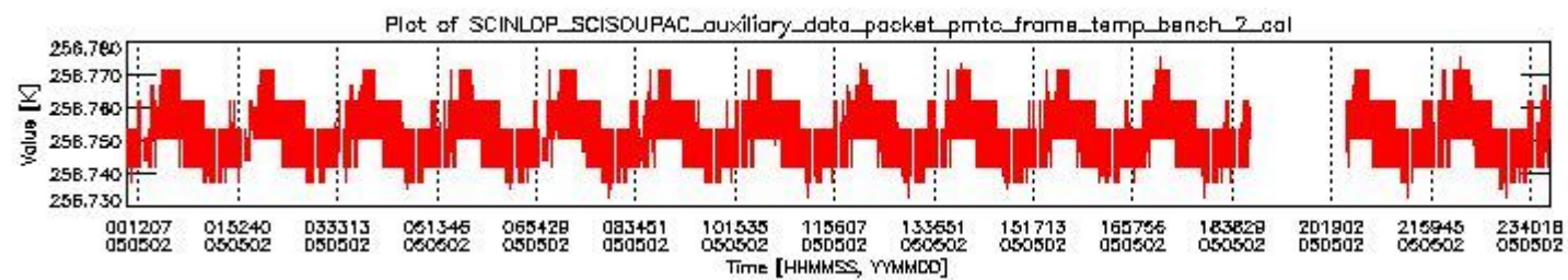
sciamachy_daily_report_level0_PFHS_5_32_N_20050502_1.PNG
