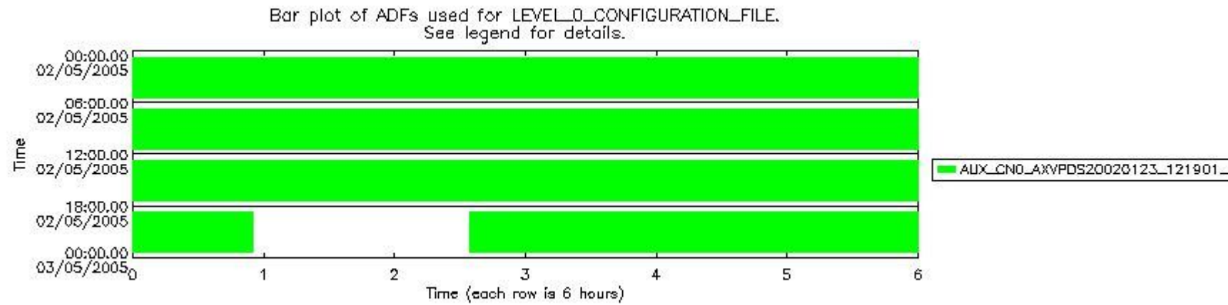
sciamachy_daily_report_level0_PFHS_5_32_N_20050502_5.PNG
