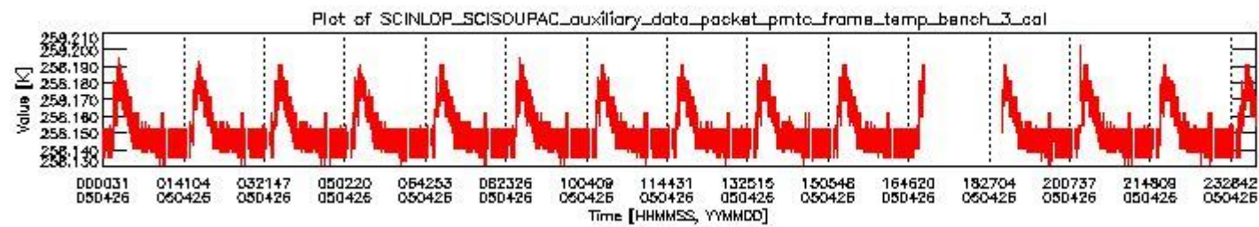
sciamachy_daily_report_level0_PFHS_5_32_N_20050426_2.PNG
