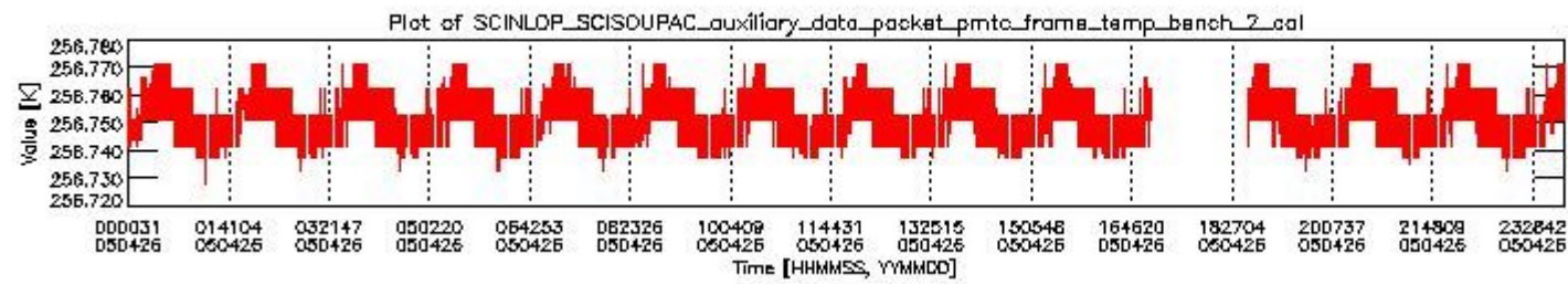
sciamachy_daily_report_level0_PFHS_5_32_N_20050426_1.PNG
