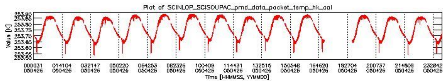
sciamachy_daily_report_level0_PFHS_5_32_N_20050426_3.PNG
