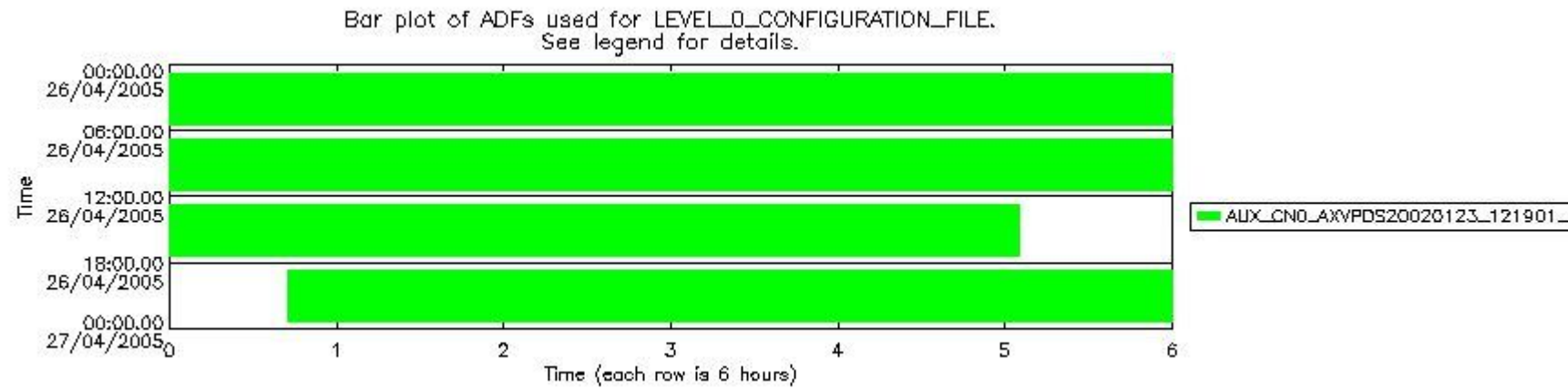
sciamachy_daily_report_level0_PFHS_5_32_N_20050426_5.PNG
