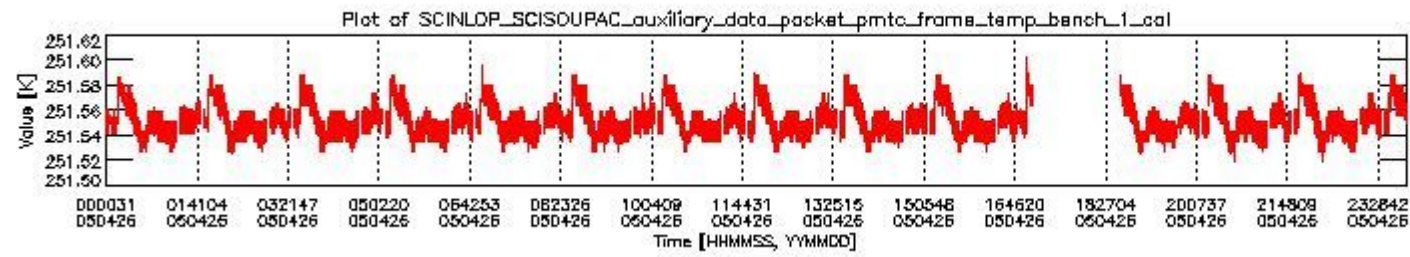
sciamachy_daily_report_level0_PFHS_5_32_N_20050426_0.PNG
