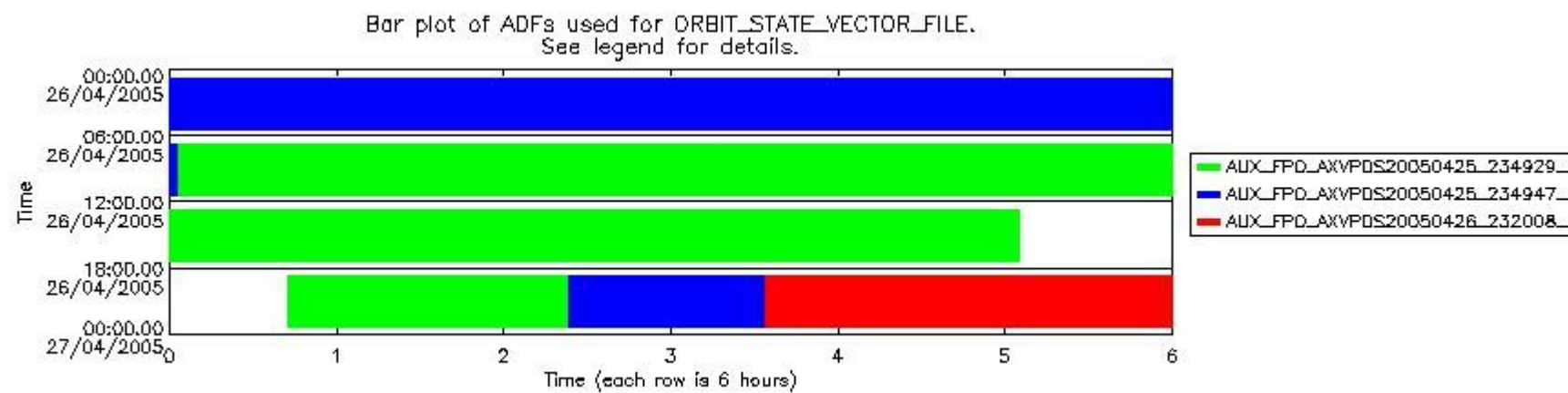
sciamachy_daily_report_level0_PFHS_5_32_N_20050426_6.PNG
