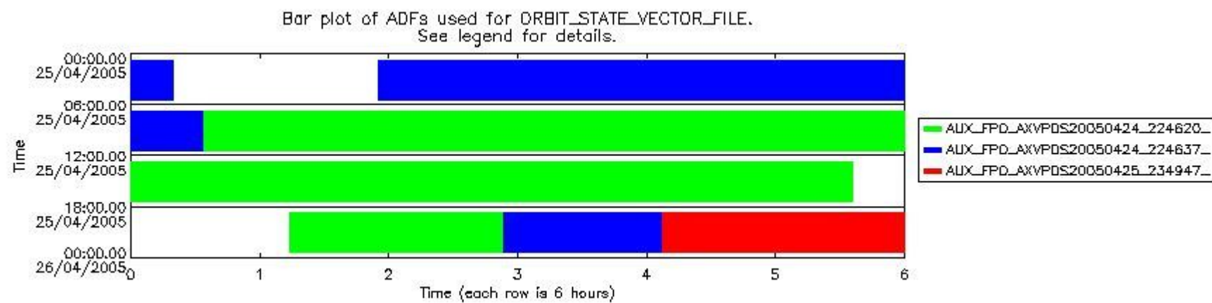
sciamachy_daily_report_level0_PFHS_5_32_N_20050425_6.PNG
