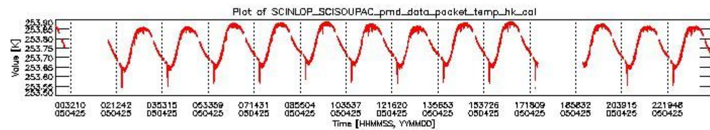
sciamachy_daily_report_level0_PFHS_5_32_N_20050425_3.PNG
