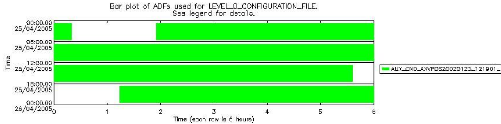
sciamachy_daily_report_level0_PFHS_5_32_N_20050425_5.PNG
