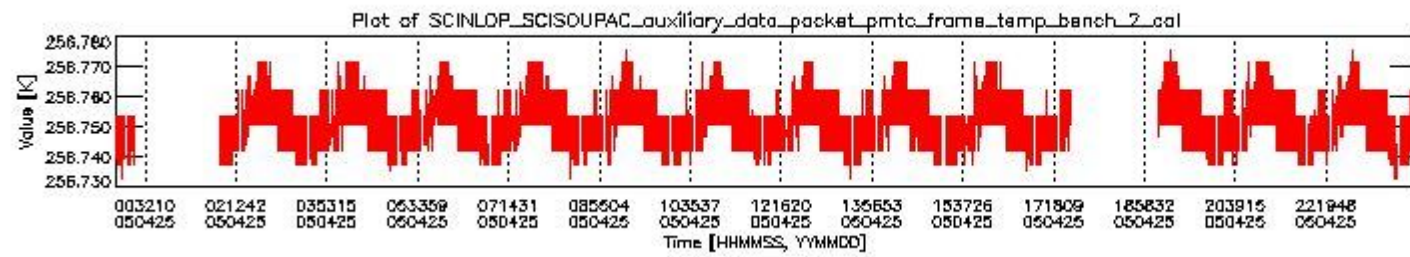
sciamachy_daily_report_level0_PFHS_5_32_N_20050425_1.PNG
