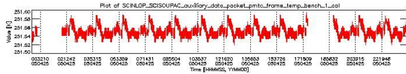
sciamachy_daily_report_level0_PFHS_5_32_N_20050425_0.PNG
