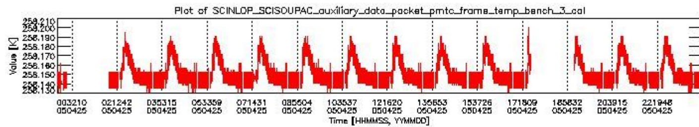
sciamachy_daily_report_level0_PFHS_5_32_N_20050425_2.PNG
