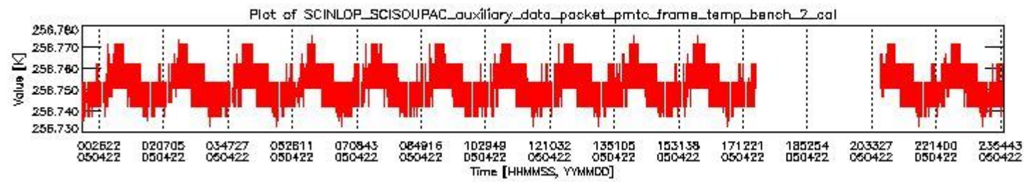
sciamachy_daily_report_level0_PFHS_5_32_N_20050422_1.PNG
