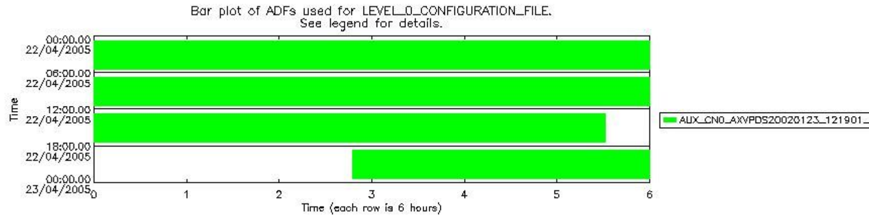
sciamachy_daily_report_level0_PFHS_5_32_N_20050422_5.PNG
