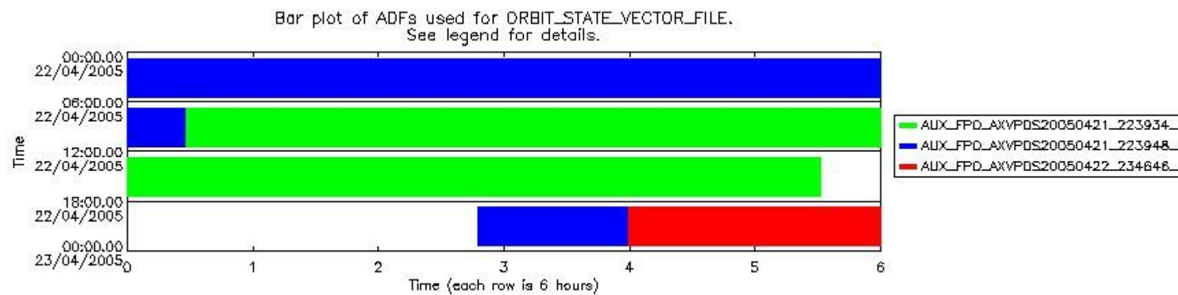
sciamachy_daily_report_level0_PFHS_5_32_N_20050422_6.PNG
