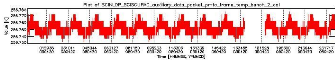
sciamachy_daily_report_level0_PFHS_5_32_N_20050420_1.PNG
