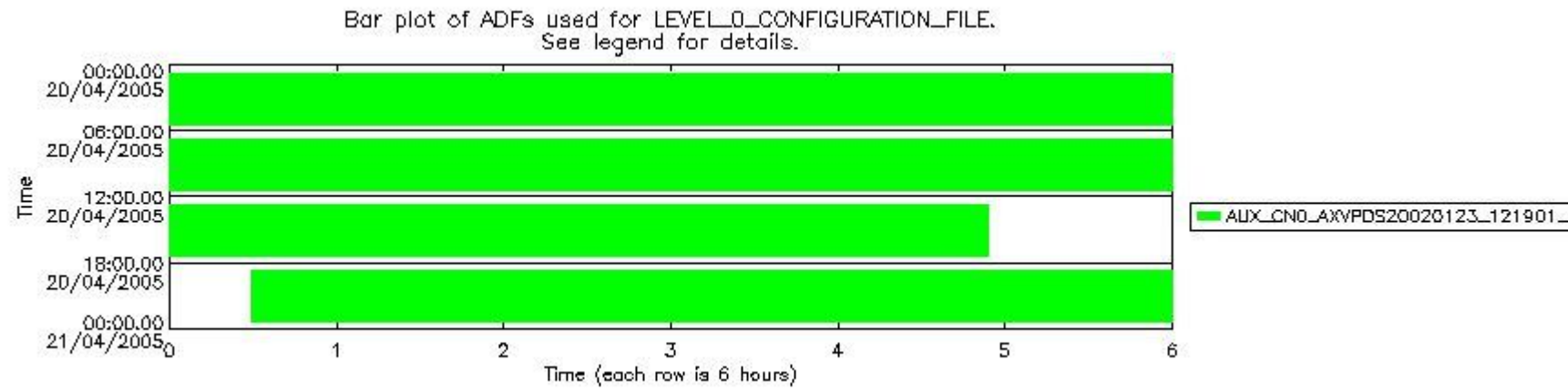
sciamachy_daily_report_level0_PFHS_5_32_N_20050420_5.PNG
