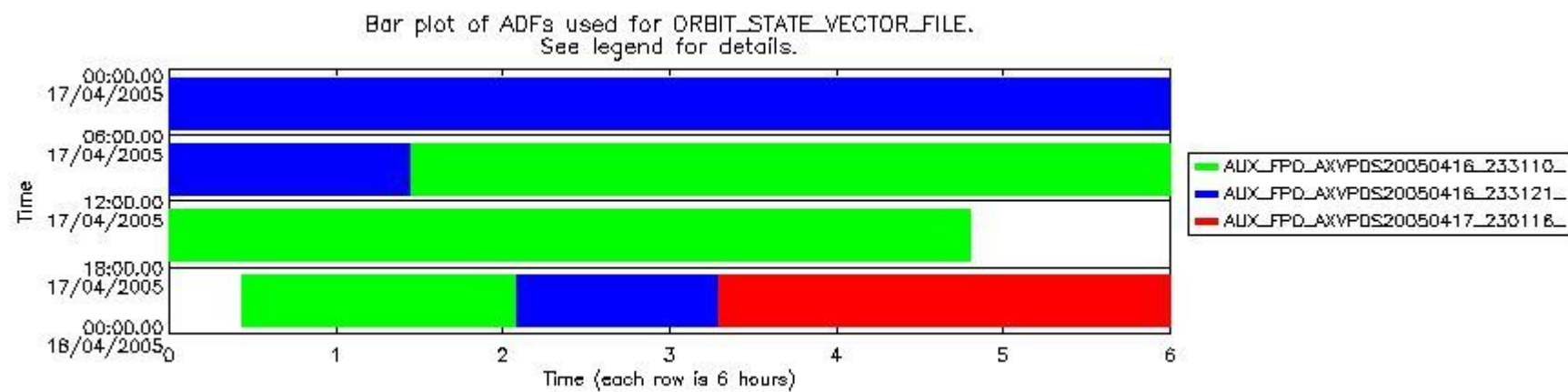
sciamachy_daily_report_level0_PFHS_5_32_N_20050417_6.PNG
