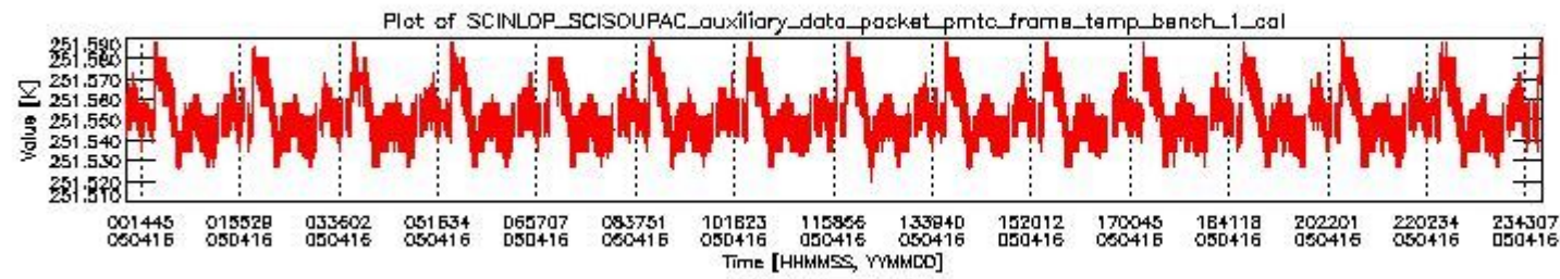
sciamachy_daily_report_level0_PFHS_5_32_N_20050416_0.PNG
