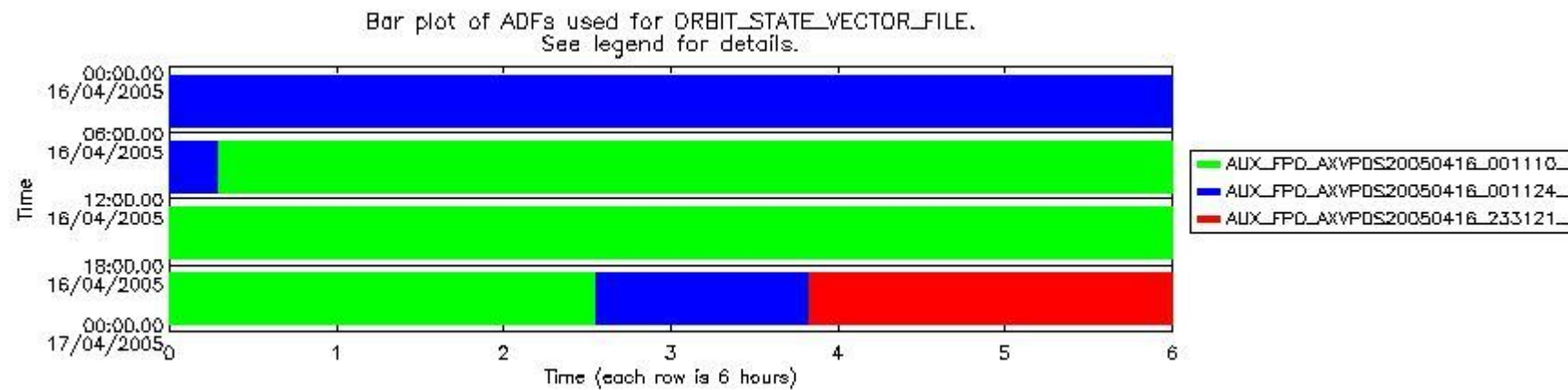
sciamachy_daily_report_level0_PFHS_5_32_N_20050416_6.PNG
