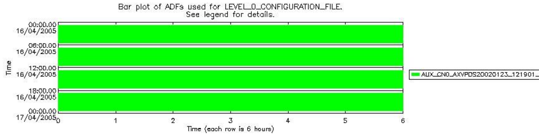
sciamachy_daily_report_level0_PFHS_5_32_N_20050416_5.PNG
