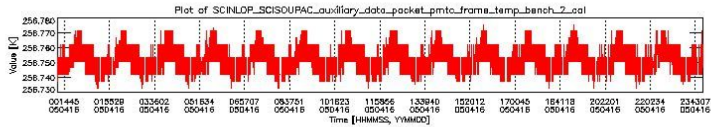
sciamachy_daily_report_level0_PFHS_5_32_N_20050416_1.PNG
