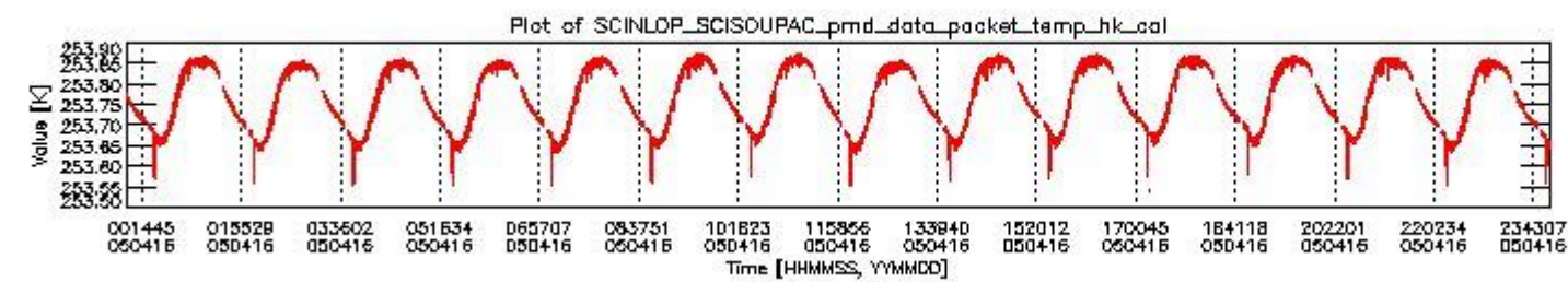
sciamachy_daily_report_level0_PFHS_5_32_N_20050416_3.PNG
