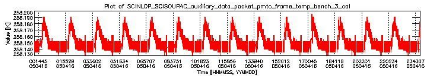
sciamachy_daily_report_level0_PFHS_5_32_N_20050416_2.PNG
