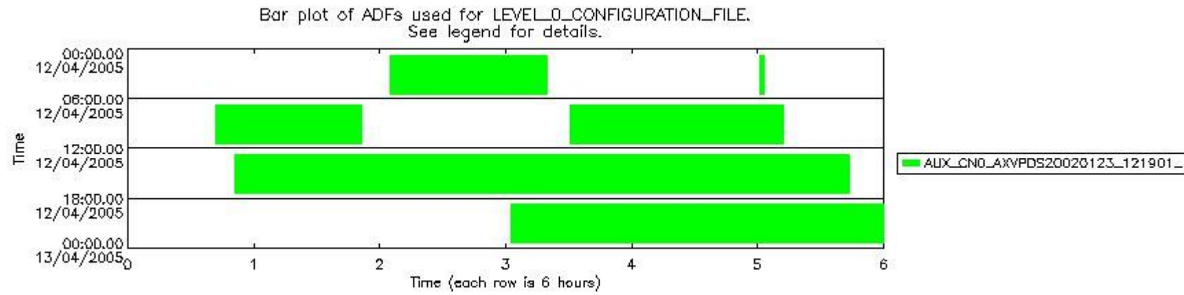
sciamachy_daily_report_level0_PFHS_5_32_N_20050412_5.PNG
