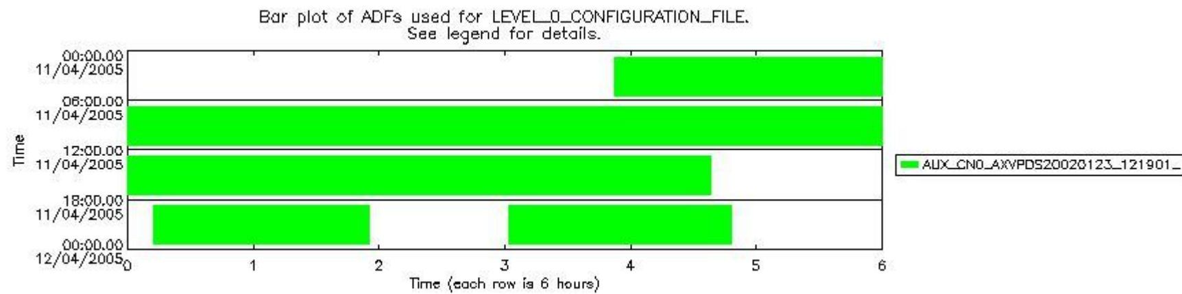
sciamachy_daily_report_level0_PFHS_5_32_N_20050411_5.PNG
