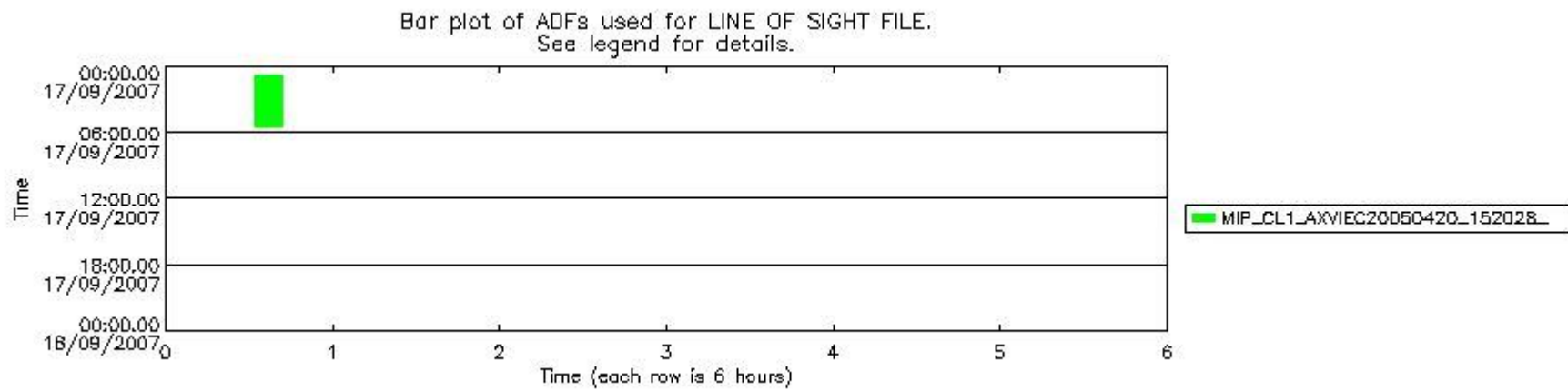
mipas_daily_report_level1_MIPAS_4_67_P_20070917_55.PNG
