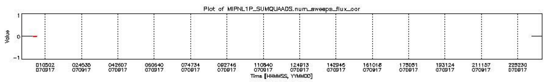
mipas_daily_report_level1_MIPAS_4_67_P_20070917_12.PNG
