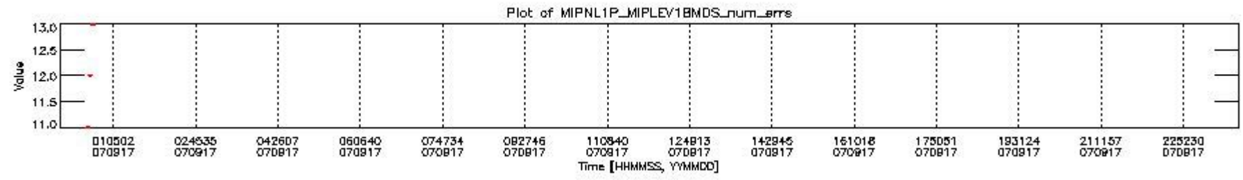
mipas_daily_report_level1_MIPAS_4_67_P_20070917_28.PNG
