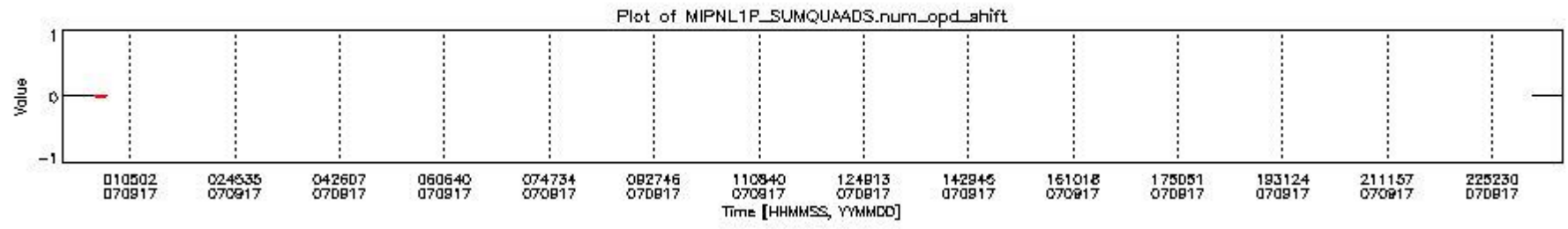
mipas_daily_report_level1_MIPAS_4_67_P_20070917_10.PNG
