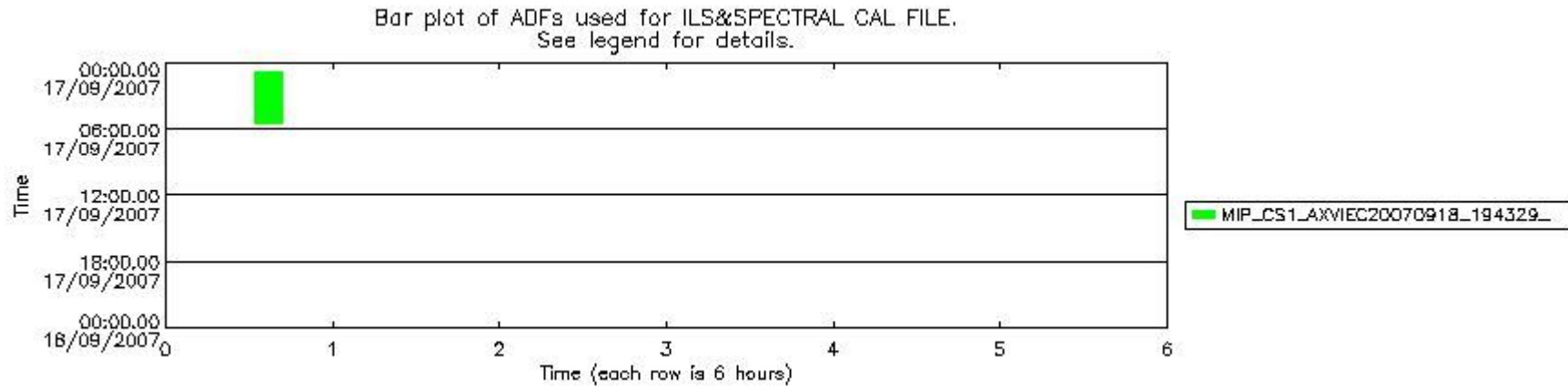
mipas_daily_report_level1_MIPAS_4_67_P_20070917_53.PNG
