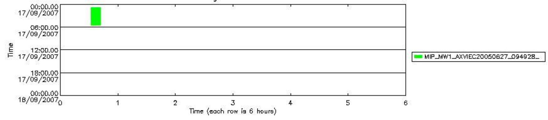
mipas_daily_report_level1_MIPAS_4_67_P_20070917_58.PNG
