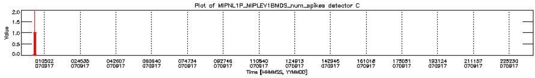
mipas_daily_report_level1_MIPAS_4_67_P_20070917_24.PNG
