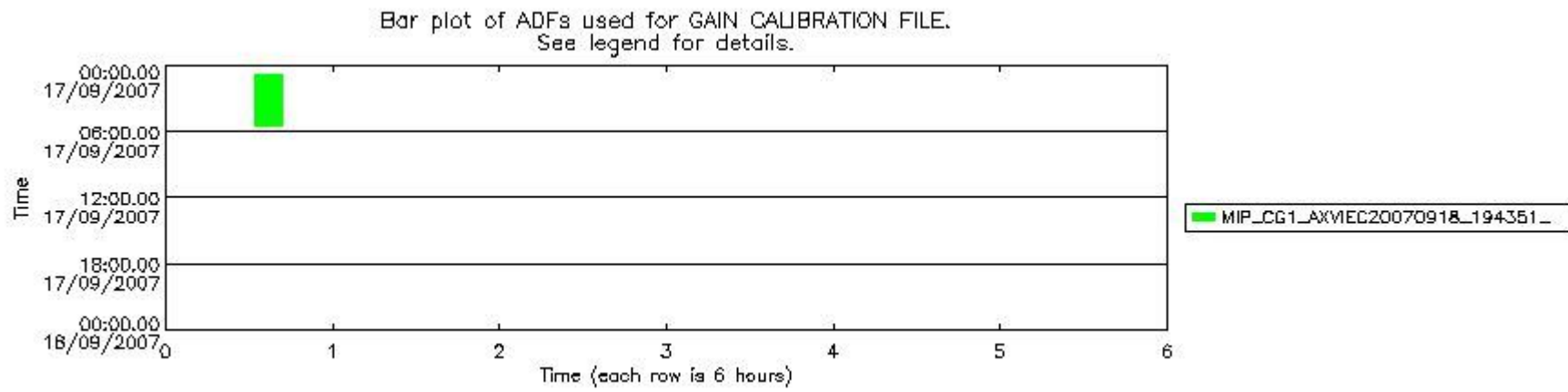
mipas_daily_report_level1_MIPAS_4_67_P_20070917_54.PNG
