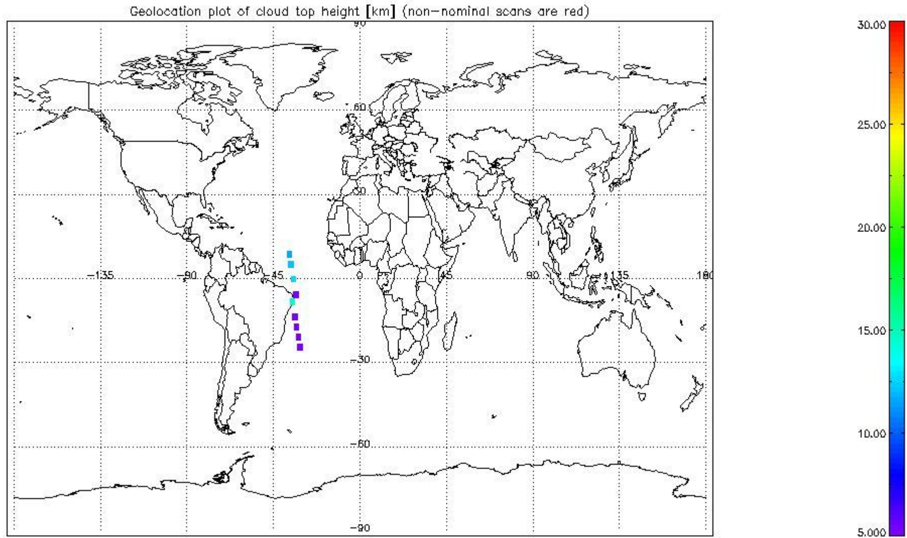
mipas_daily_report_level1_MIPAS_4_67_P_20070917_51.PNG
