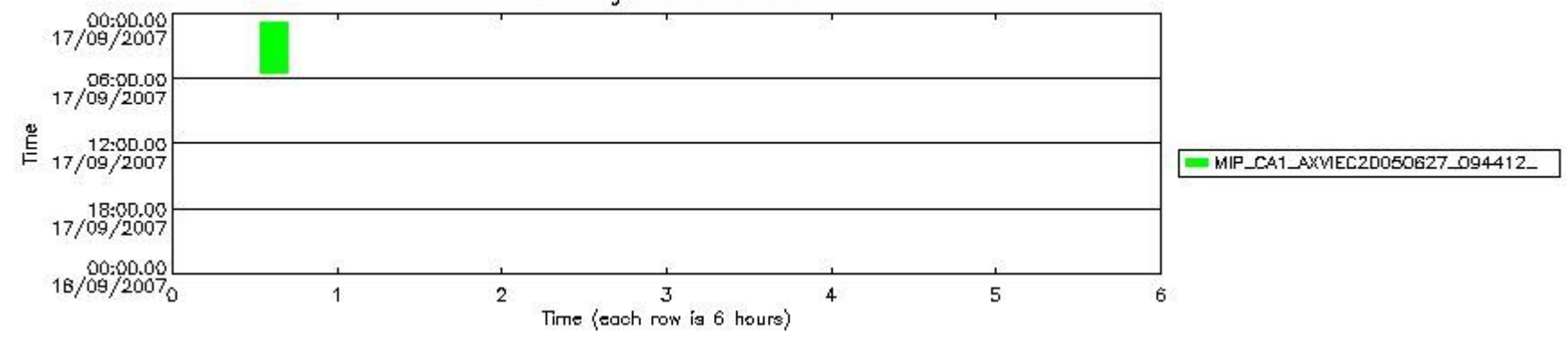
mipas_daily_report_level1_MIPAS_4_67_P_20070917_56.PNG
