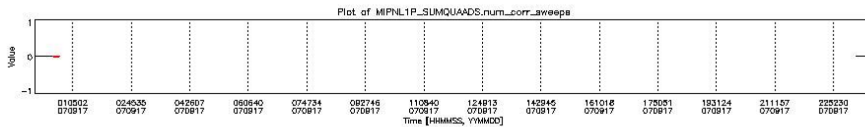
mipas_daily_report_level1_MIPAS_4_67_P_20070917_2.PNG
