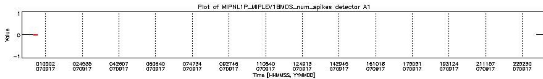
mipas_daily_report_level1_MIPAS_4_67_P_20070917_16.PNG
