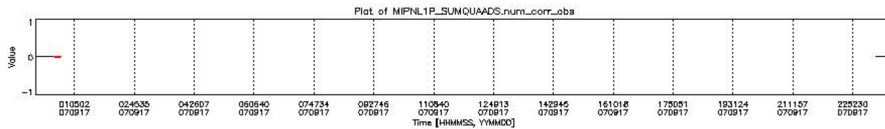
mipas_daily_report_level1_MIPAS_4_67_P_20070917_6.PNG
