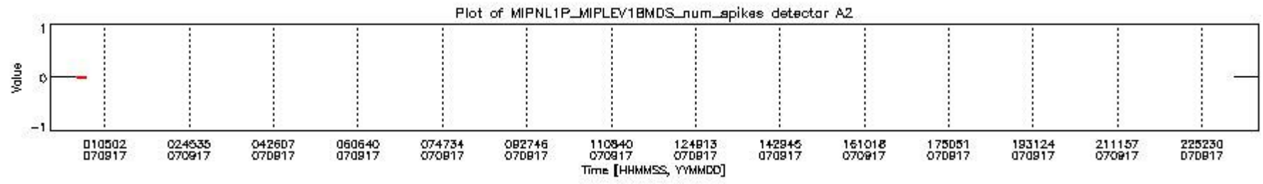
mipas_daily_report_level1_MIPAS_4_67_P_20070917_18.PNG
