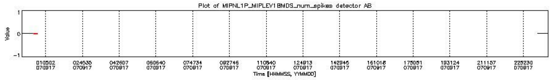
mipas_daily_report_level1_MIPAS_4_67_P_20070917_20.PNG
