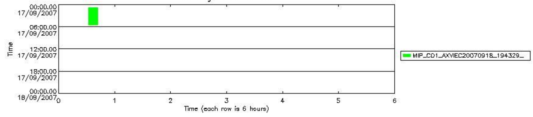
mipas_daily_report_level1_MIPAS_4_67_P_20070917_57.PNG
