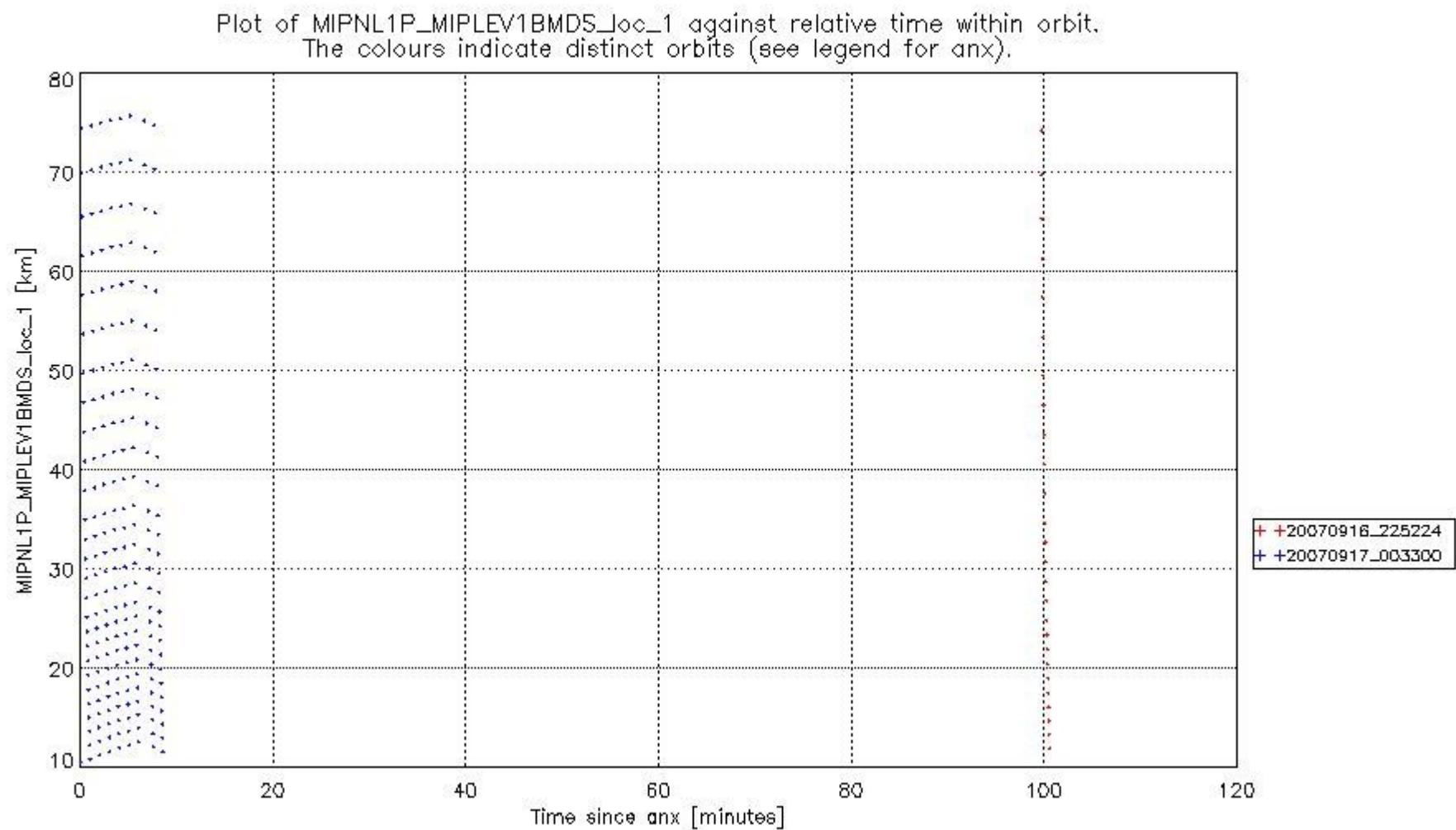
mipas_daily_report_level1_MIPAS_4_67_P_20070917_50.PNG
