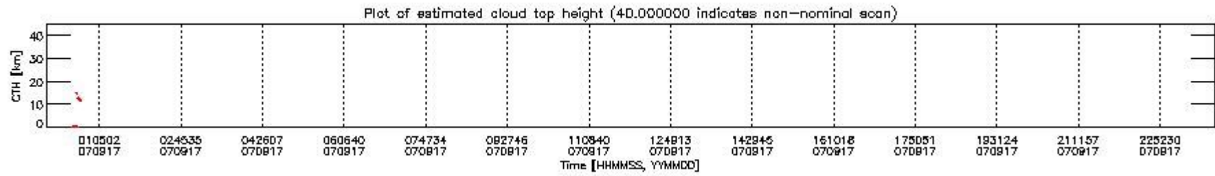
mipas_daily_report_level1_MIPAS_4_67_P_20070917_51.PNG
