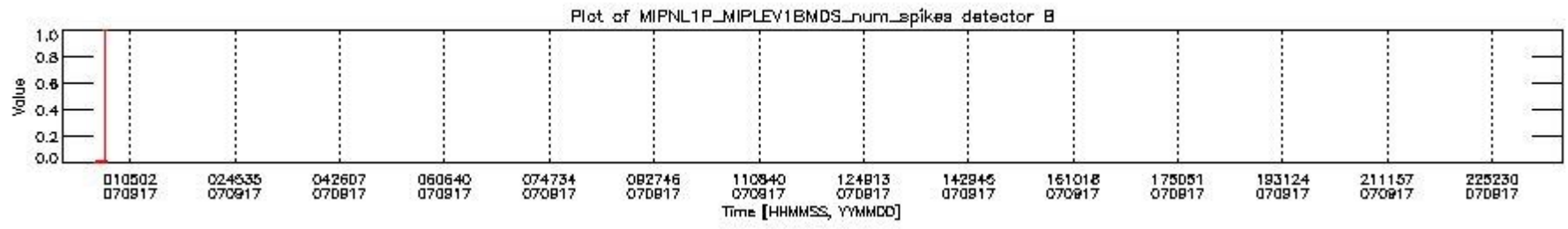
mipas_daily_report_level1_MIPAS_4_67_P_20070917_22.PNG
