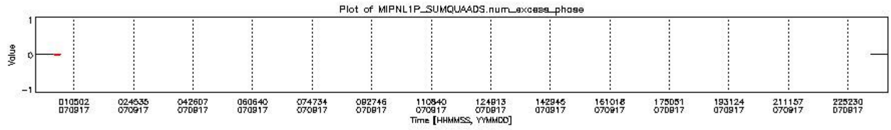
mipas_daily_report_level1_MIPAS_4_67_P_20070917_8.PNG
