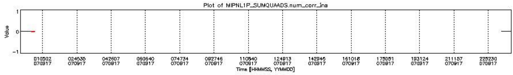
mipas_daily_report_level1_MIPAS_4_67_P_20070917_4.PNG
