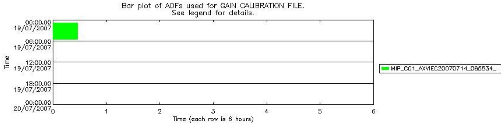
mipas_daily_report_level1_OFL_MIPAS_4_67_P_20070719_54.PNG
