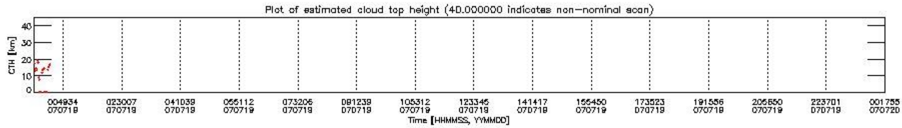
mipas_daily_report_level1_OFL_MIPAS_4_67_P_20070719_51.PNG
