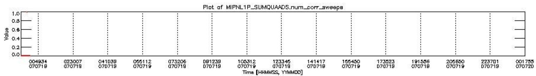
mipas_daily_report_level1_OFL_MIPAS_4_67_P_20070719_2.PNG
