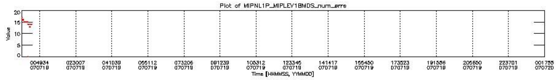
mipas_daily_report_level1_OFL_MIPAS_4_67_P_20070719_28.PNG
