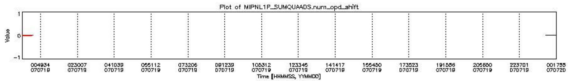
mipas_daily_report_level1_OFL_MIPAS_4_67_P_20070719_10.PNG
