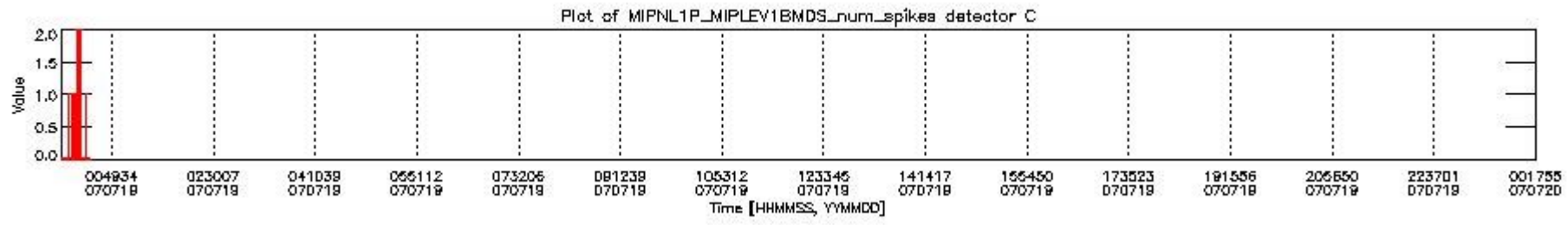
mipas_daily_report_level1_OFL_MIPAS_4_67_P_20070719_24.PNG
