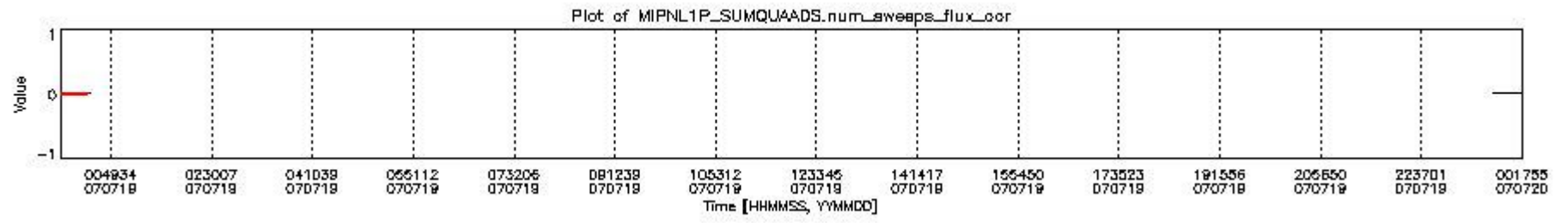
mipas_daily_report_level1_OFL_MIPAS_4_67_P_20070719_12.PNG
