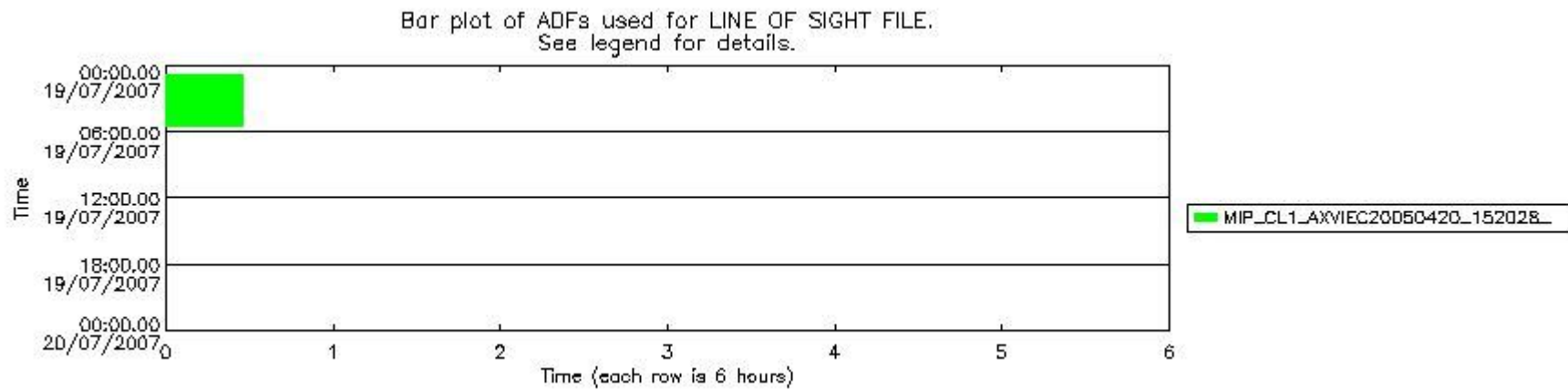
mipas_daily_report_level1_OFL_MIPAS_4_67_P_20070719_55.PNG
