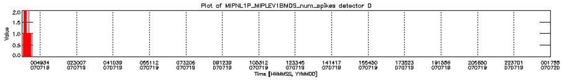
mipas_daily_report_level1_OFL_MIPAS_4_67_P_20070719_26.PNG
