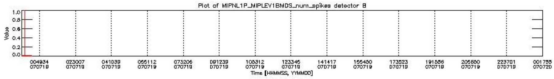
mipas_daily_report_level1_OFL_MIPAS_4_67_P_20070719_22.PNG
