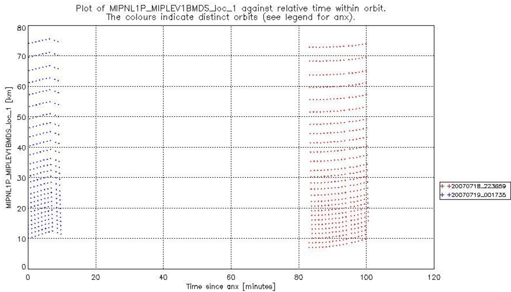
mipas_daily_report_level1_OFL_MIPAS_4_67_P_20070719_50.PNG
