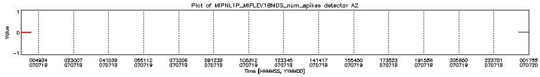
mipas_daily_report_level1_OFL_MIPAS_4_67_P_20070719_18.PNG
