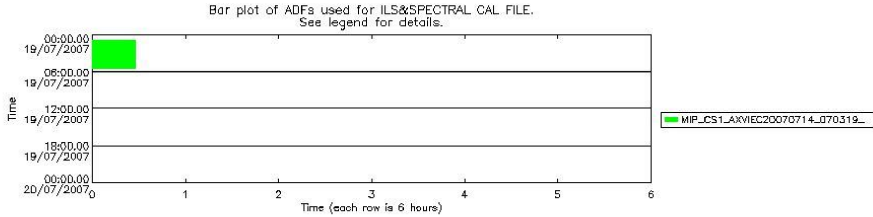
mipas_daily_report_level1_OFL_MIPAS_4_67_P_20070719_53.PNG
