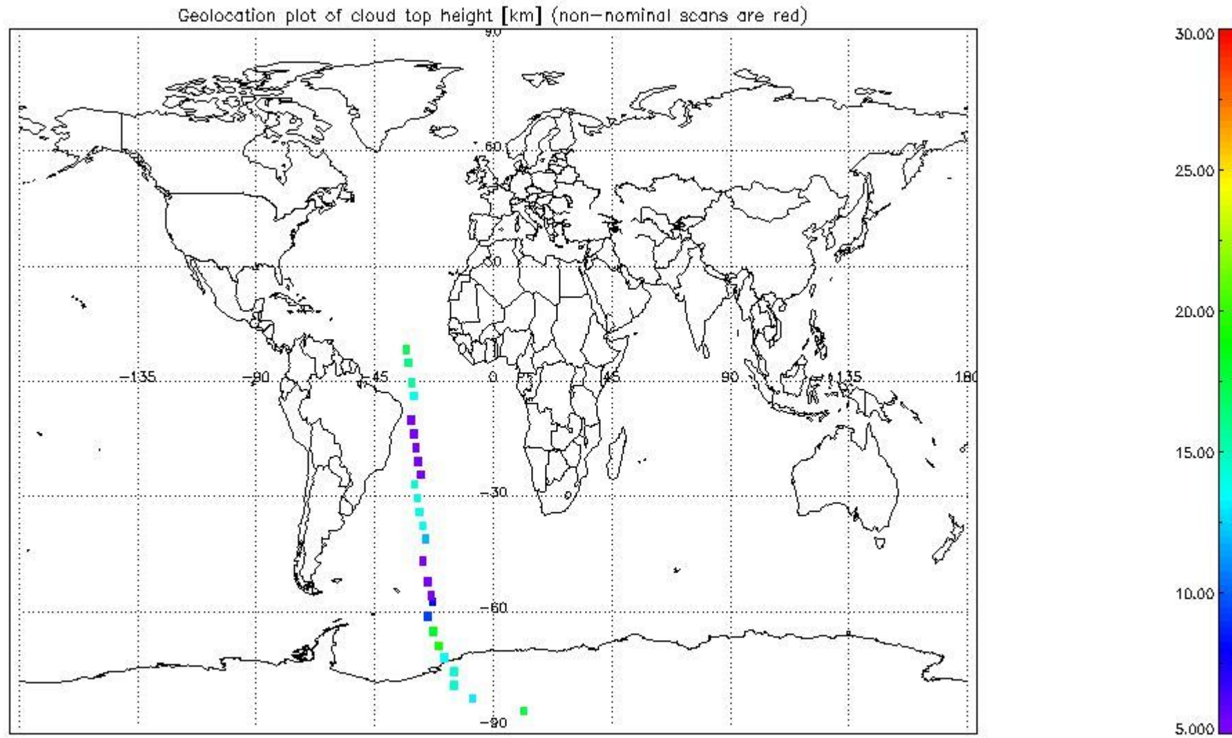
mipas_daily_report_level1_OFL_MIPAS_4_67_P_20070719_51.PNG
