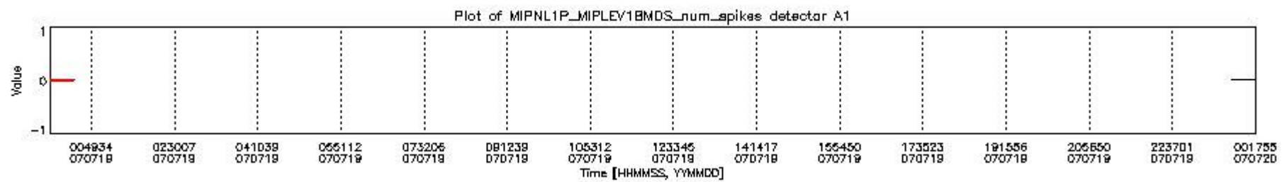
mipas_daily_report_level1_OFL_MIPAS_4_67_P_20070719_16.PNG
