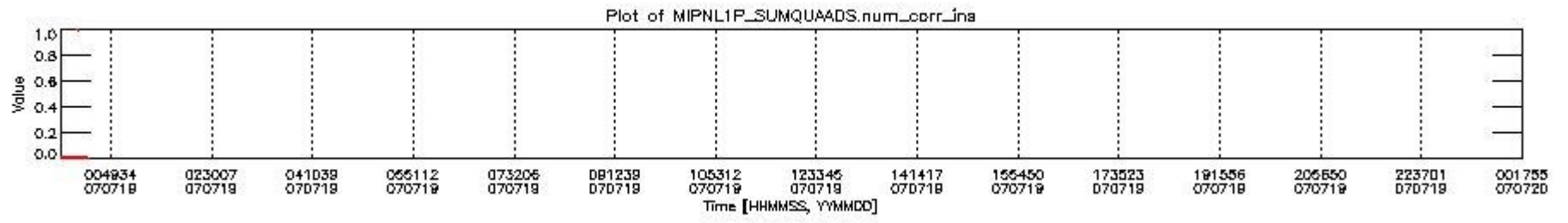
mipas_daily_report_level1_OFI_MIPAS_4_67_P_20070719_4.PNG
