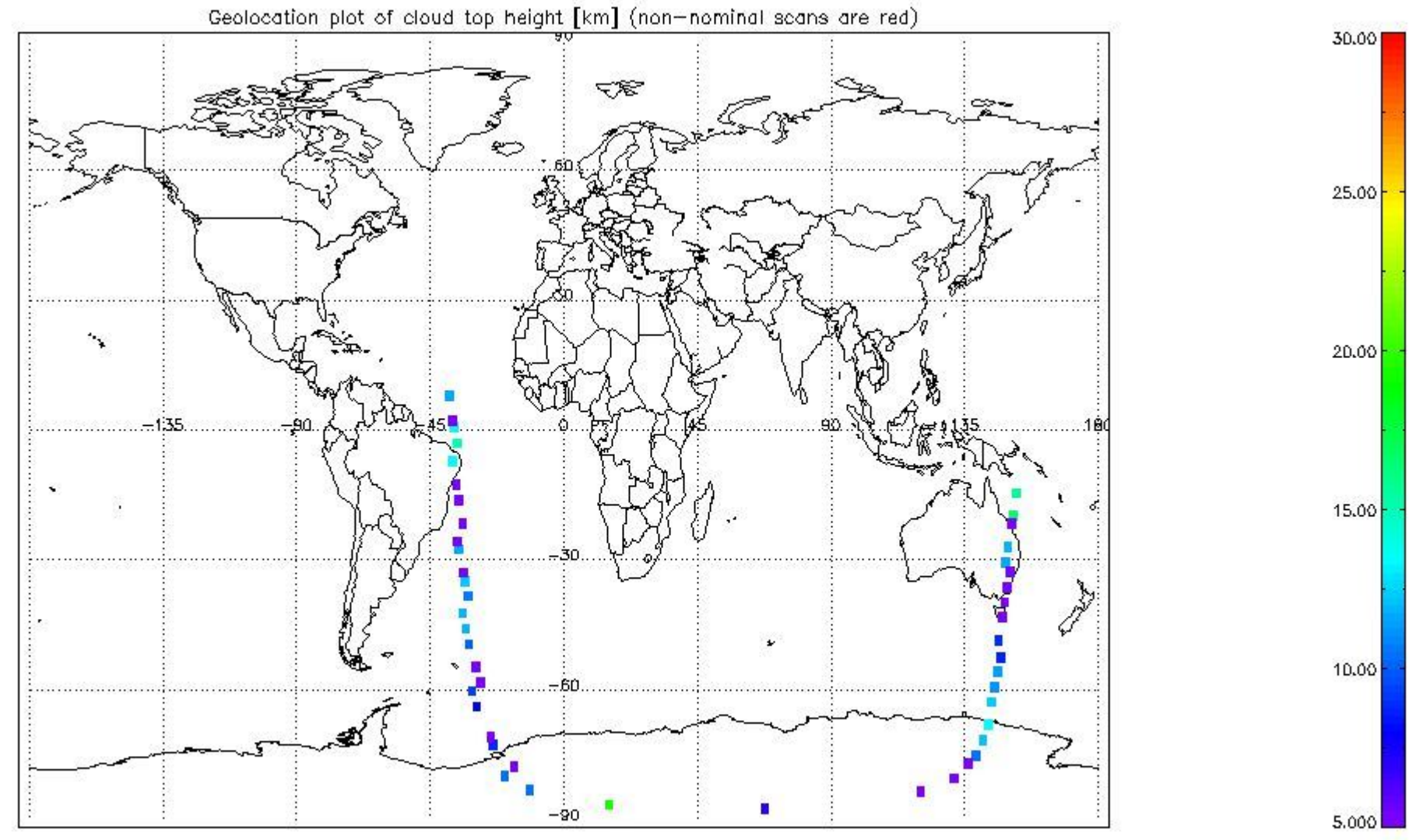
mipas_daily_report_level1_OFL_MIPAS_4_67_P_20070522_51.PNG
