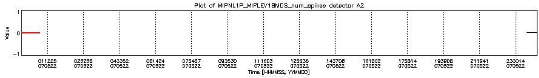
mipas_daily_report_level1_OFI_MIPAS_4_67_P_20070522_18.PNG
