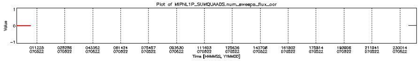
mipas_daily_report_level1_OFI_MIPAS_4_67_P_20070522_12.PNG
