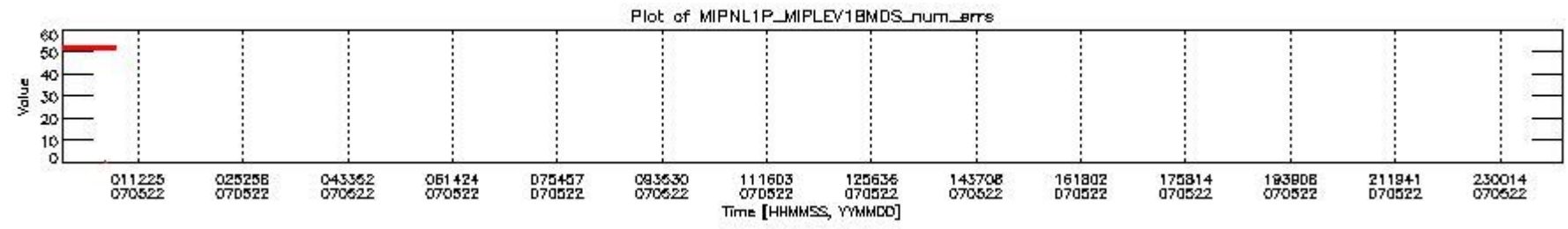
mipas_daily_report_level1_OFI_MIPAS_4_67_P_20070522_28.PNG
