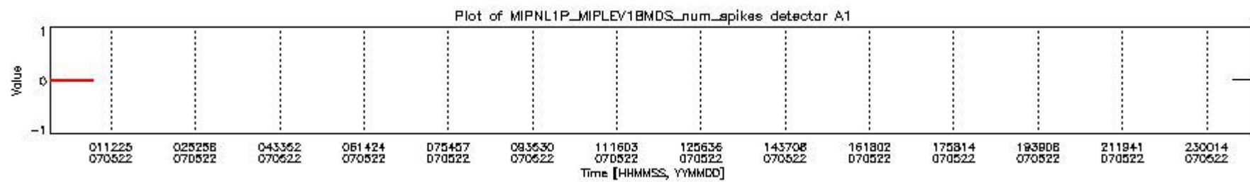
mipas_daily_report_level1_OFL_MIPAS_4_67_P_20070522_16.PNG
