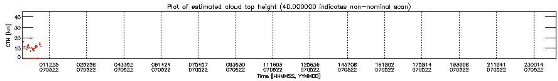
mipas_daily_report_level1_OFL_MIPAS_4_67_P_20070522_51.PNG
