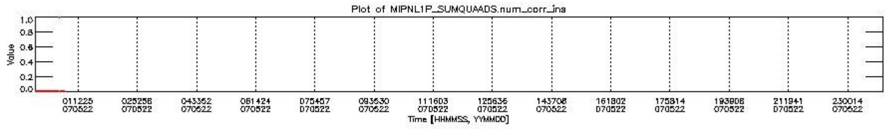
mipas_daily_report_level1_OFI_MIPAS_4_67_P_20070522_4.PNG
