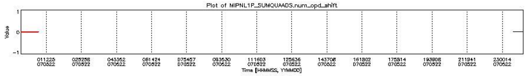
mipas_daily_report_level1_OFI_MIPAS_4_67_P_20070522_10.PNG
