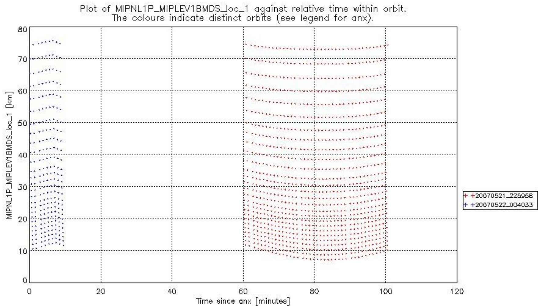
mipas_daily_report_level1_OFL_MIPAS_4_67_P_20070522_50.PNG
