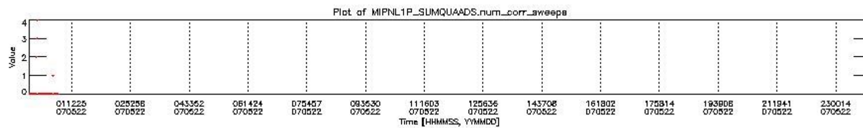
mipas_daily_report_level1_OFL_MIPAS_4_67_P_20070522_2.PNG
