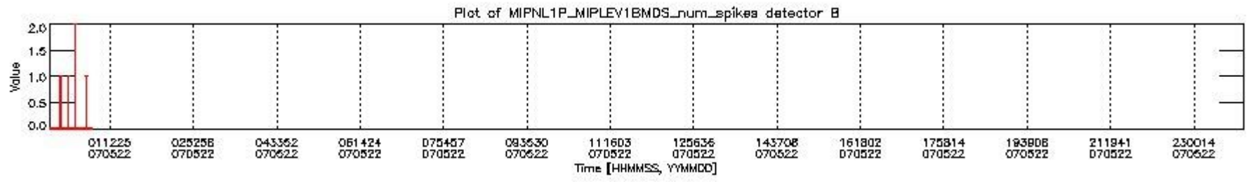
mipas_daily_report_level1_OFL_MIPAS_4_67_P_20070522_22.PNG
