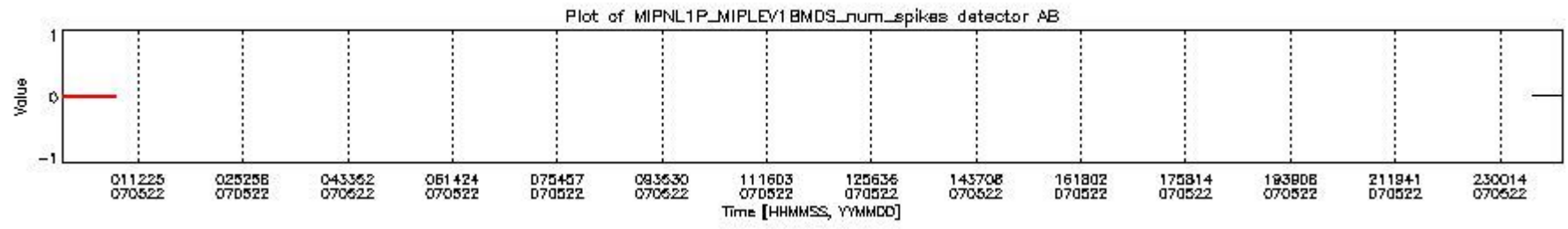
mipas_daily_report_level1_OFI_MIPAS_4_67_P_20070522_20.PNG
