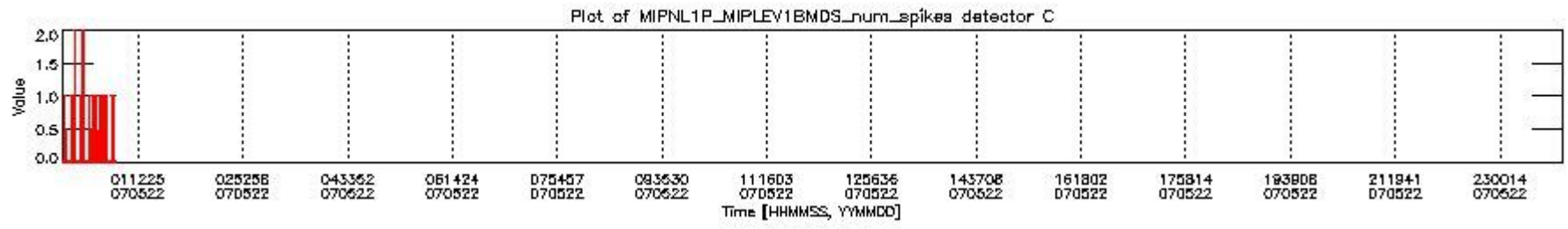
mipas_daily_report_level1_OFL_MIPAS_4_67_P_20070522_24.PNG
